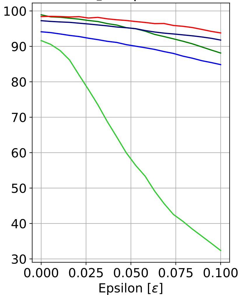
L_2 DeepFool
