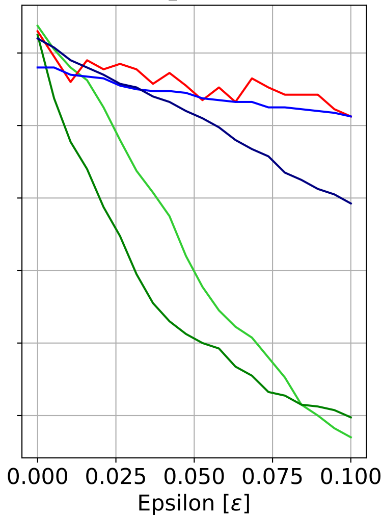
L_2 PGD
