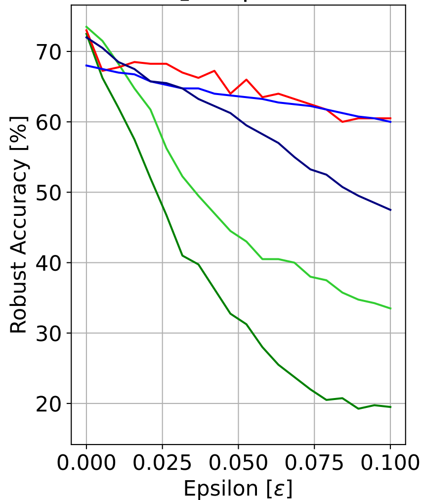
L_2 DeepFool
