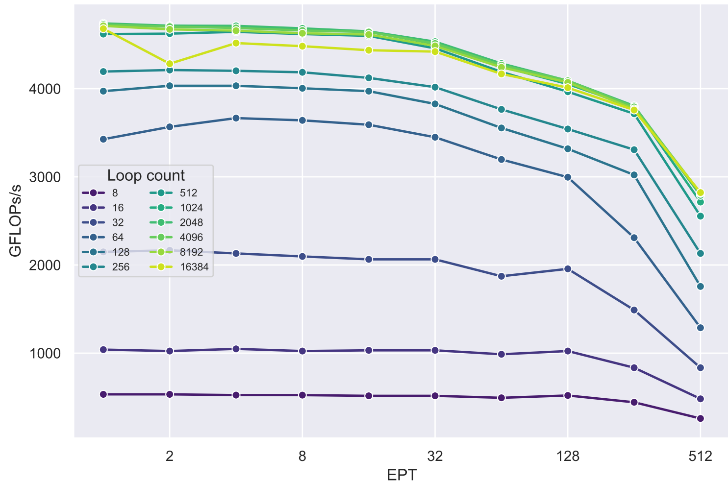
Kernel: add
