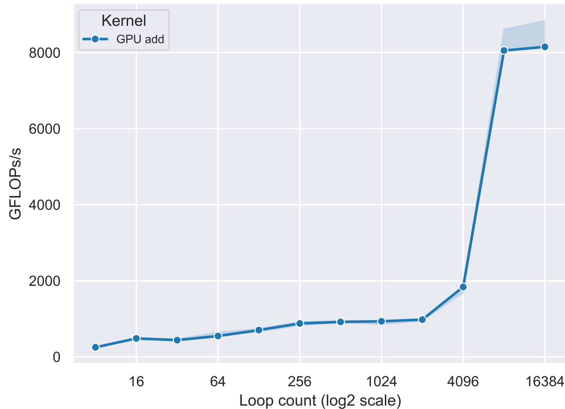
GFLOPs/s vs loop count
