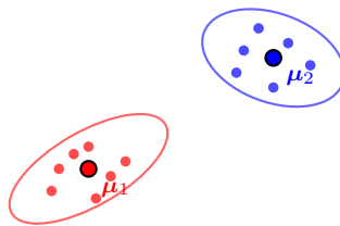
Ellipses de covariance du GMM
