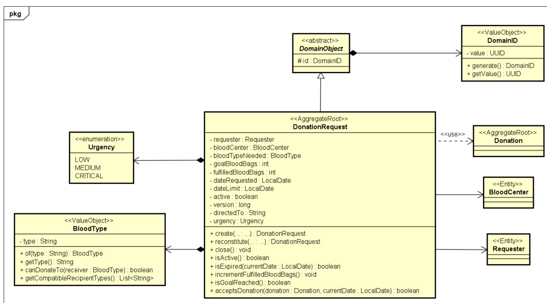
Figura 11 – Diagrama de implementação: agregado DonationRequest
