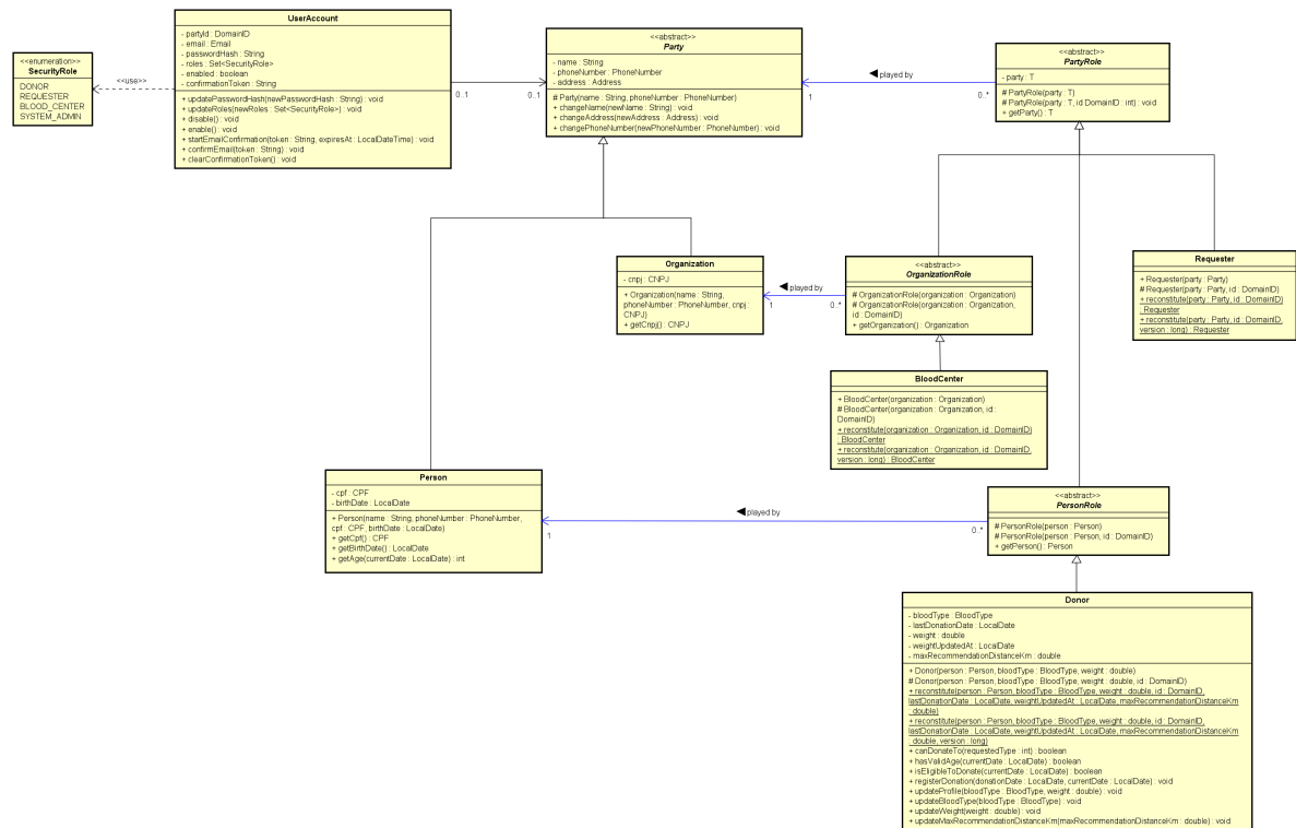
Figura 10 – Diagrama de implementação: participantes, papéis e controle de acesso
