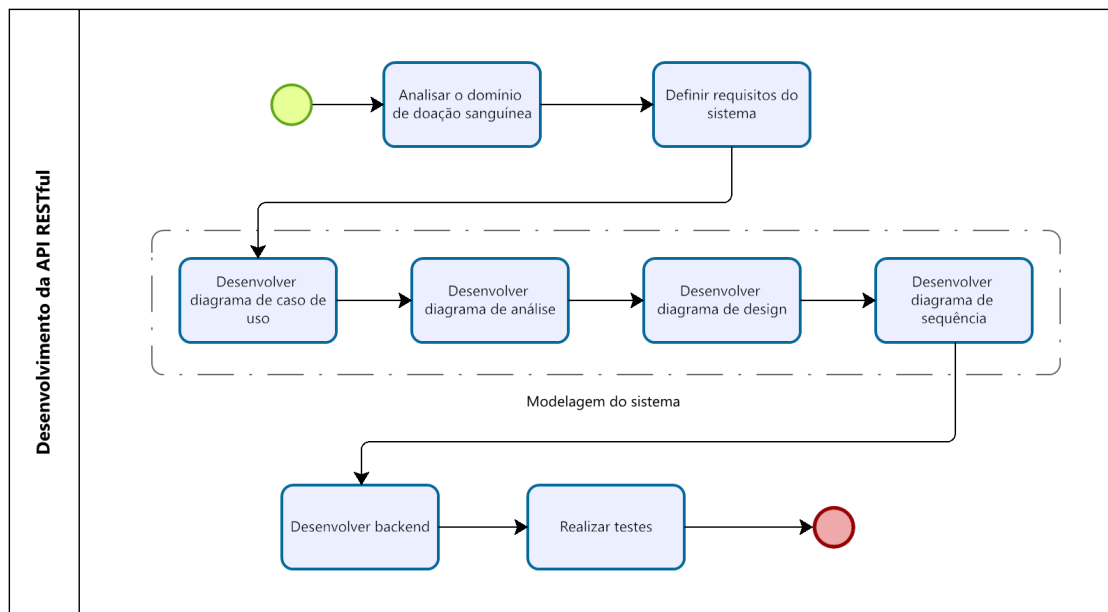
Figura 4 – Diagrama de processos do Desenvolvimento da API
