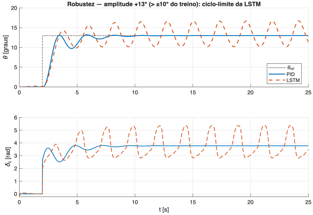
Figura 15: Pedido de 13° (acima dos 10° que a rede viu no treino): o controlador clássico (azul) acomoda limpo; a rede neural (laranja) fica oscilando sem parar.
