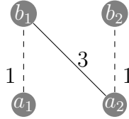
2. ábra: Maximális összsúlyú és teljes párosítás probléma
