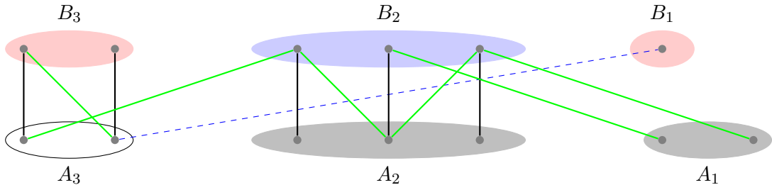
3. ábra: Magyar módszer helyessége
