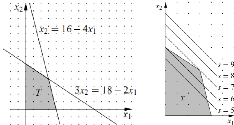
4. ábra: Kétváltozós feladat grafikus megoldása
