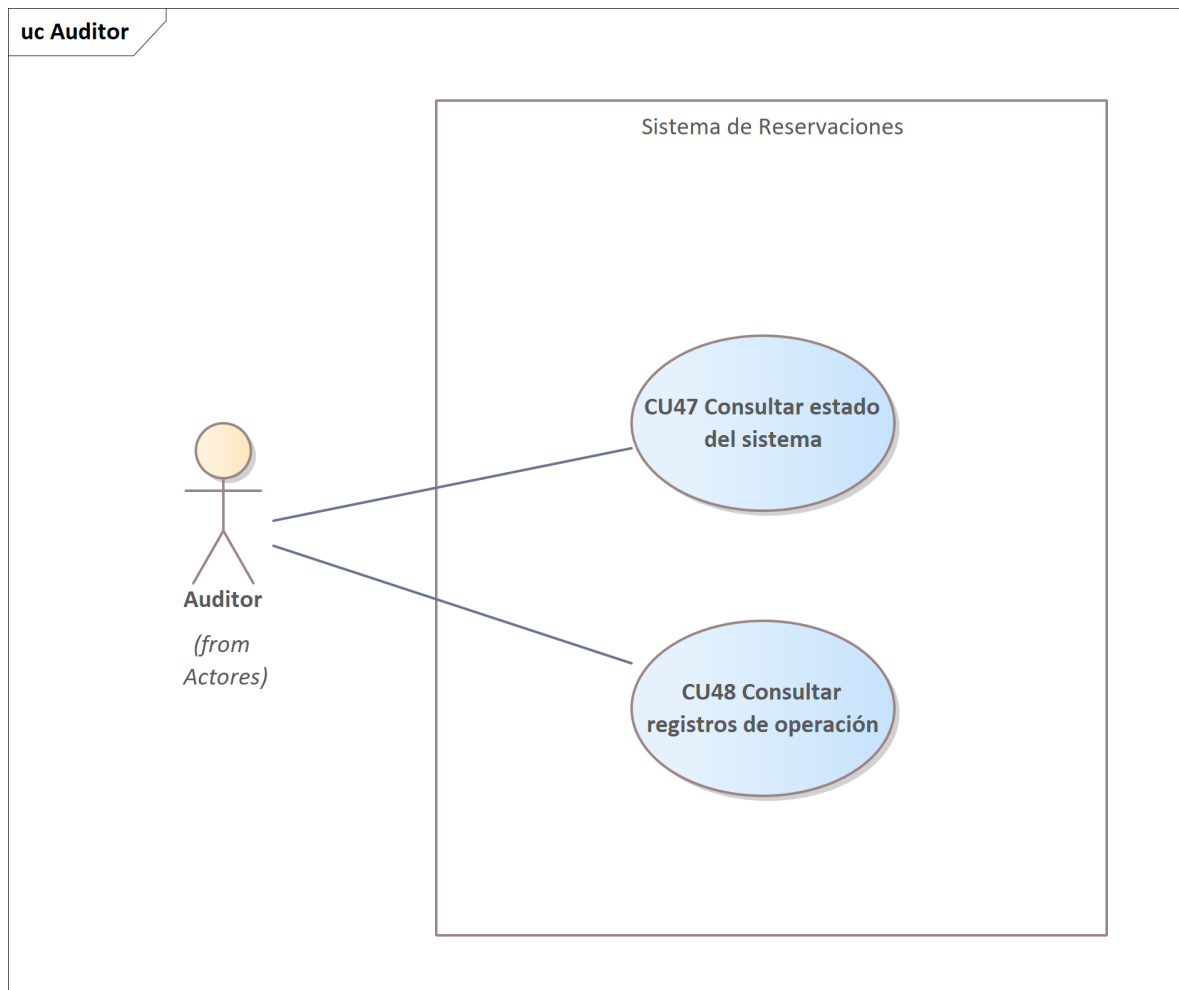
Figura 3. Diagrama de casos de uso de Auditor
