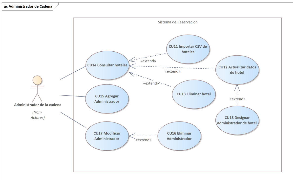
Figura 4. Diagrama de casos de uso de Administrador de cadena
