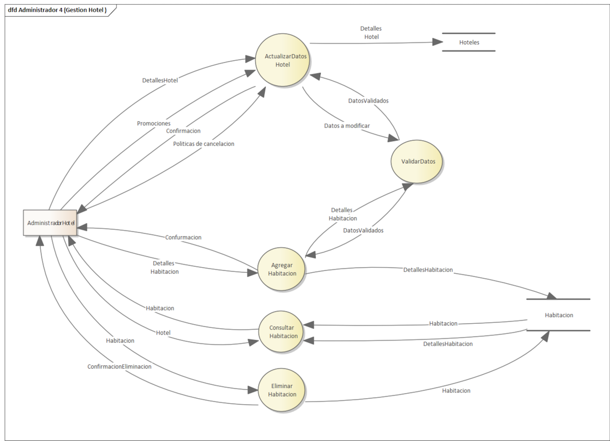
Figura 8. DFD Administrador N4 (Gestión Hotel)
