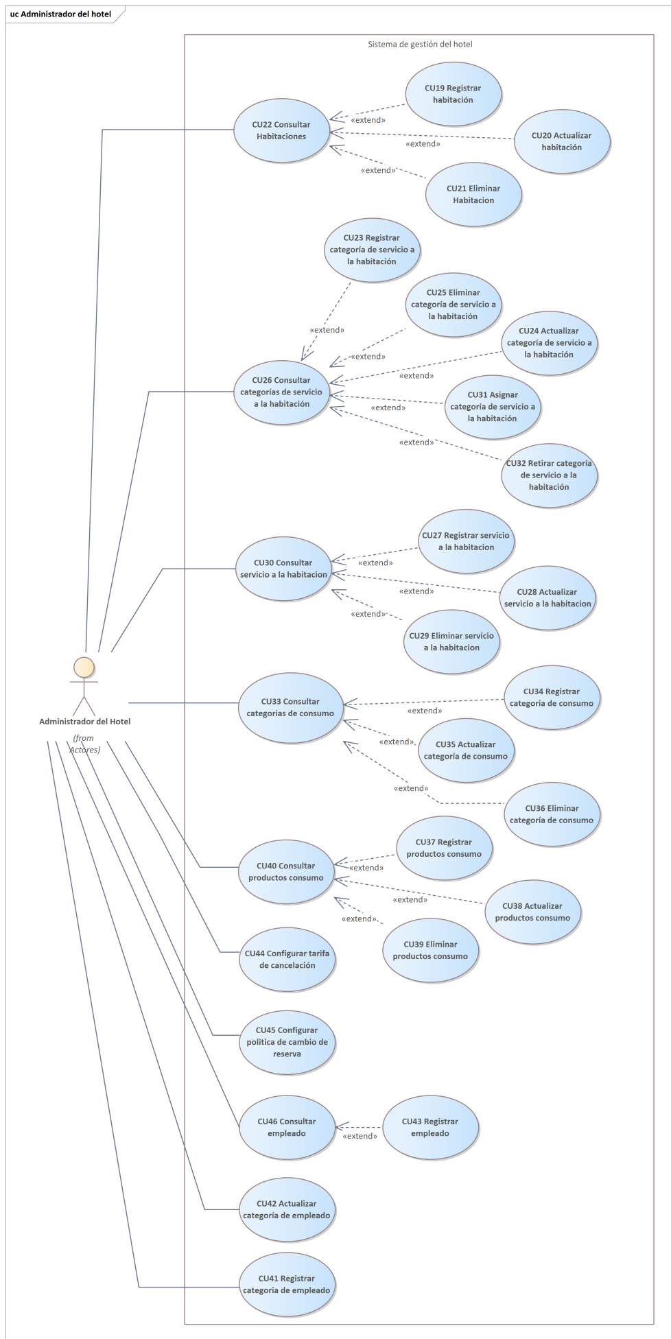
Figura 5. Diagrama de casos de uso de Administrador de hotel
