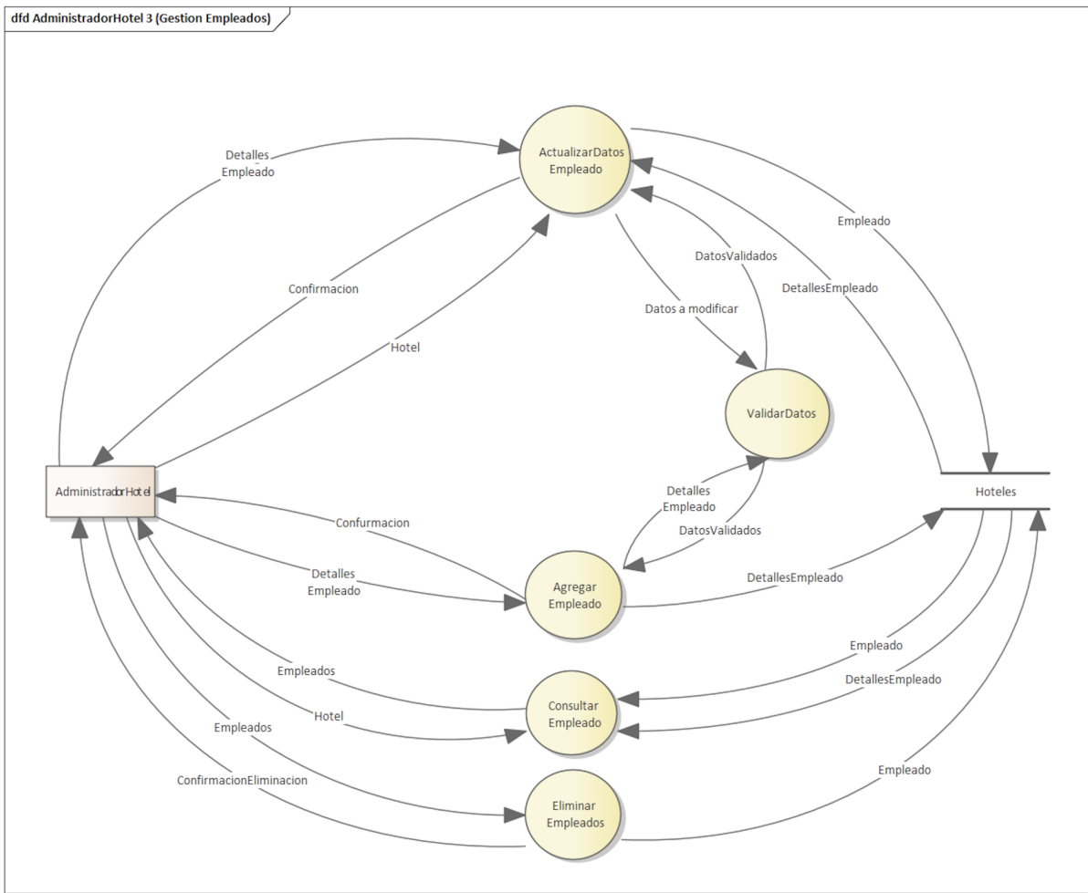
Figura 11. DFD AdministradorHotel N3 (Gestión Empleados)
