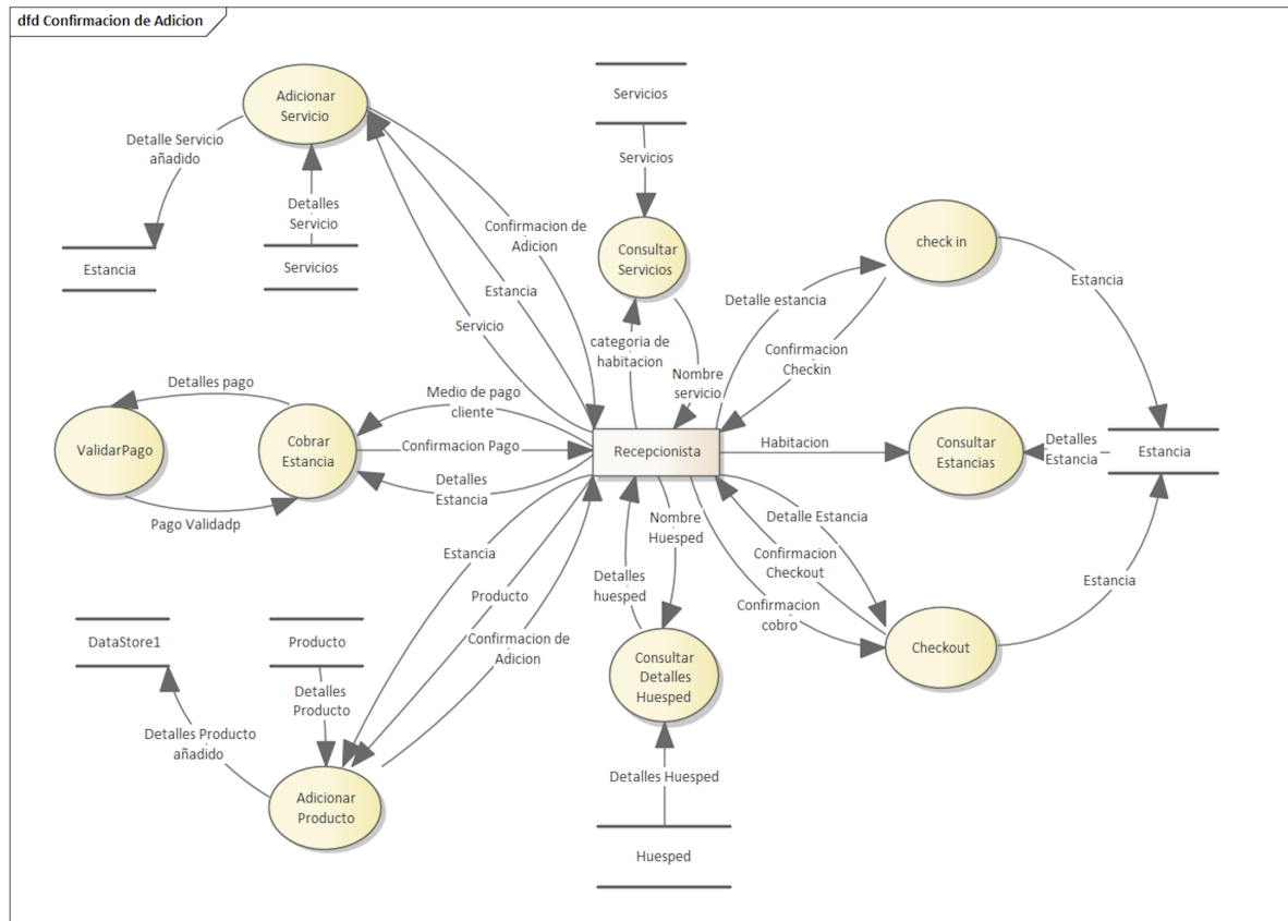
Figura 13. Diagrama de flujo de datos del Recepcionista
