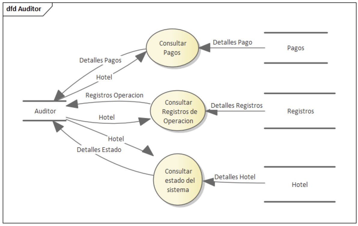
Figura 14. Diagrama de flujo de datos del Auditor
