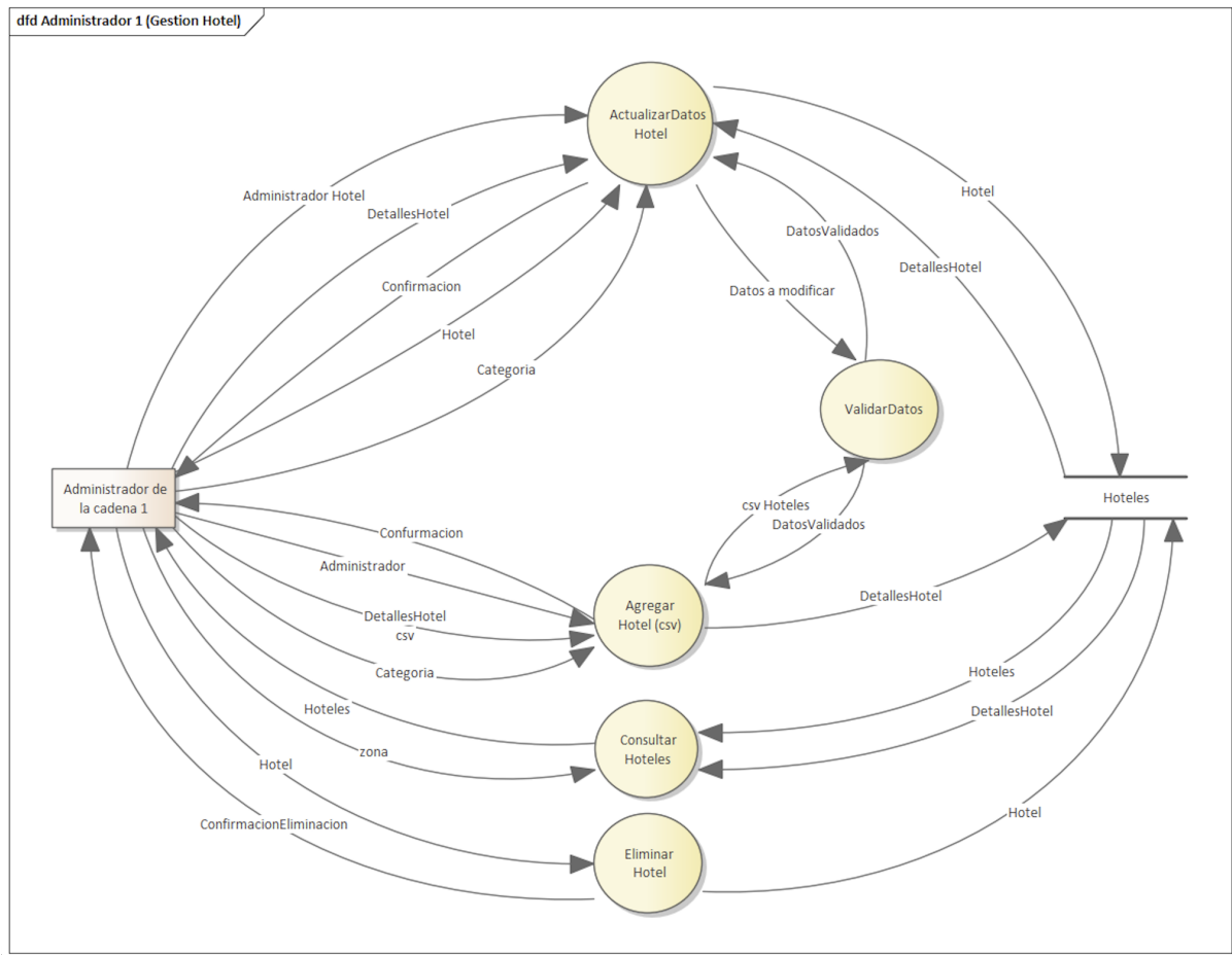
Figura 6. DFD Administrador N1 (Gestión Hotel)
