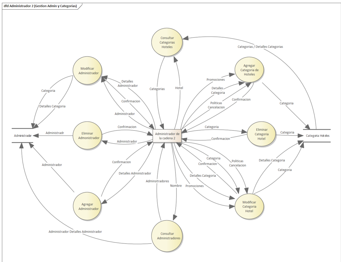
Figura 7. DFD Administrador N2 (Gestión Admin y Categorías)
