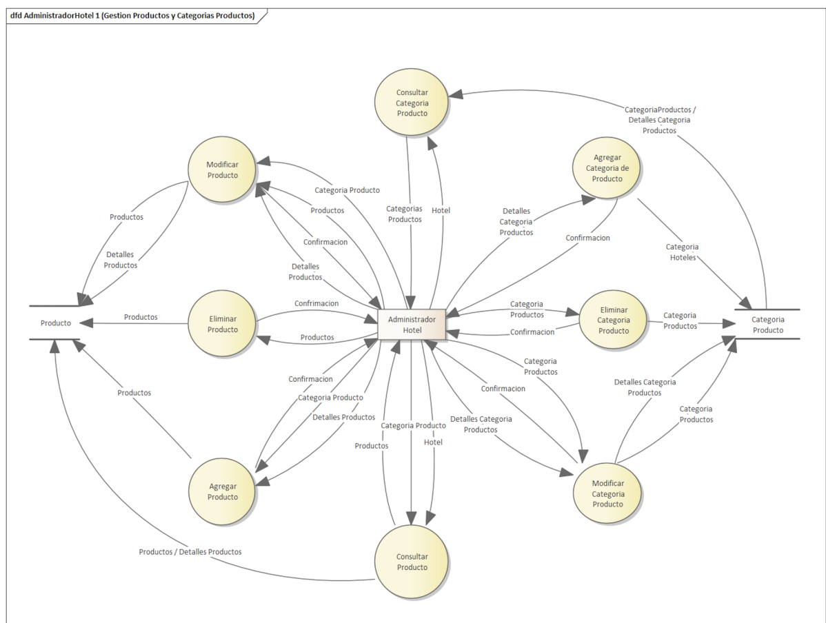
Figura 9. DFD AdministradorHotel N1 (Gestión Productos y Categorías de Productos)
