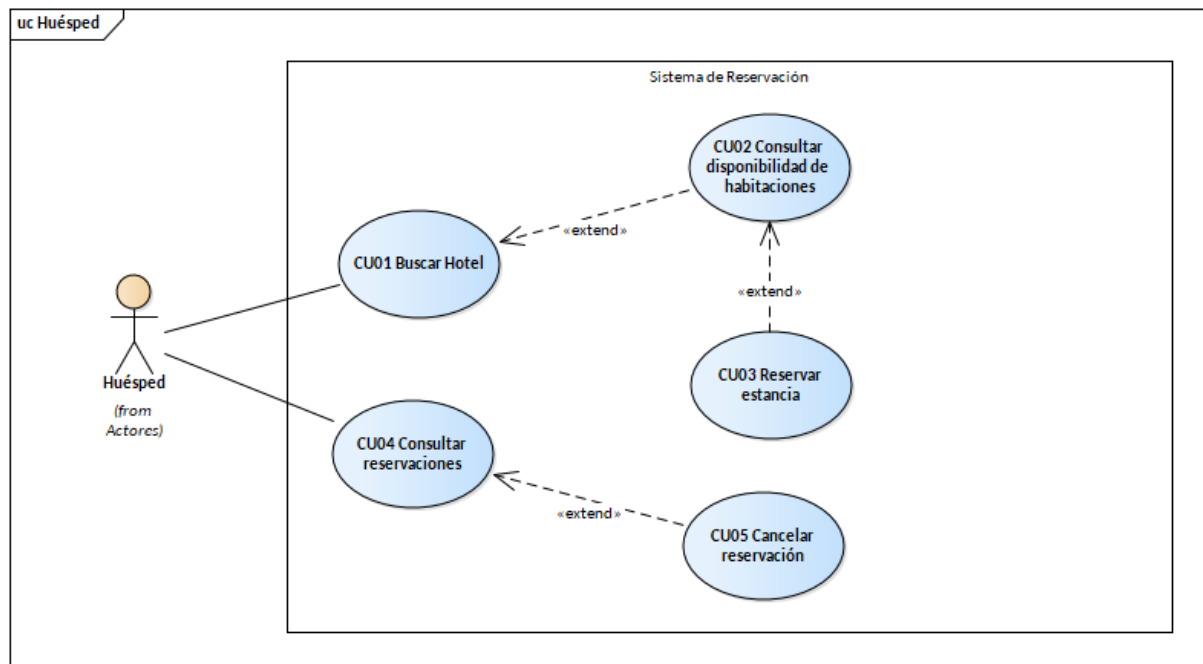
Figura 1. Diagrama de casos de uso del Huesped
