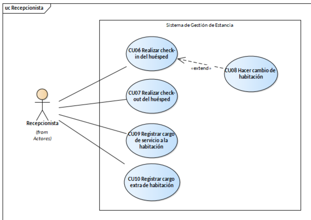
Figura 2. Diagrama de casos de uso del Recepcionista
