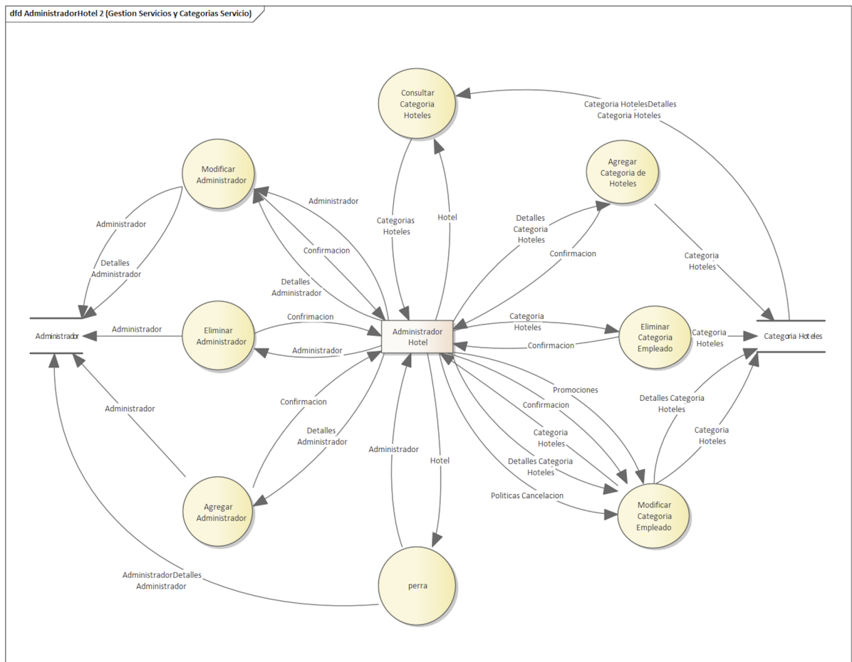
Figura 10. DFD AdministradorHotel N2 (Gestión Servicios y Categorías de Servicio)
