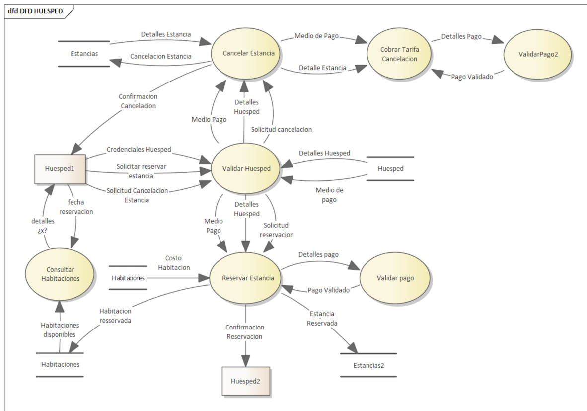
Figura 12. Diagrama de flujo de datos del Huésped
