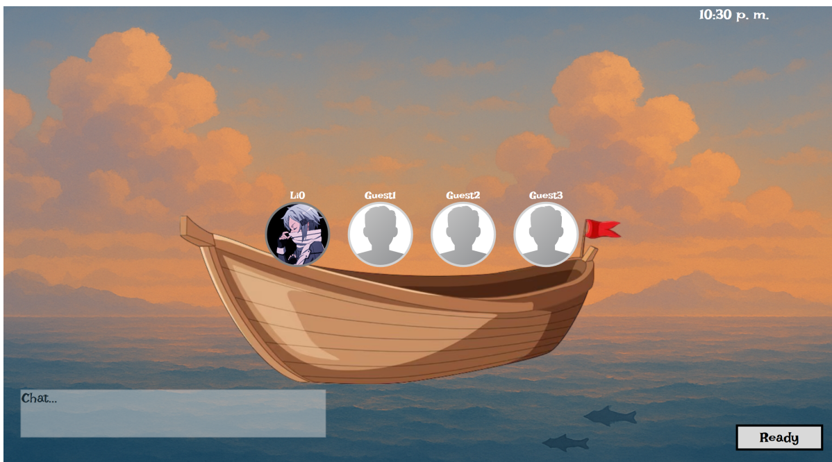
Figura 1. Lobby loggeado
