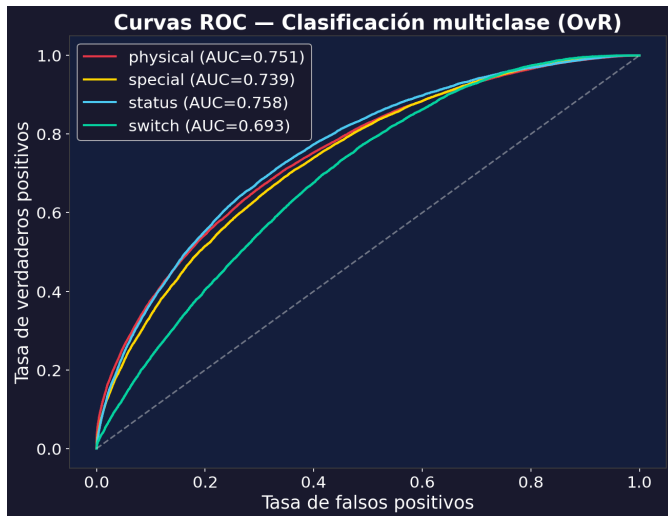
Fig. 8: Curvas ROC por clase (modelo sin switch_rate). switch es ahora la clase más difícil (AUC 0.693): el comportamiento de cambio no es predecible desde el perfil estadístico de los equipos.
