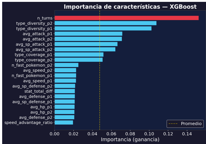
Fig. 6: Importancia de características por contribución al conjunto.
