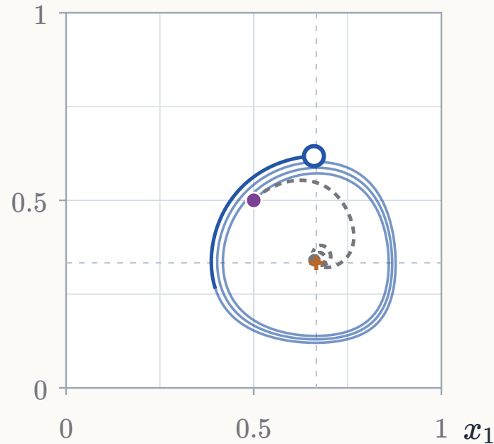
y_1 MWU
