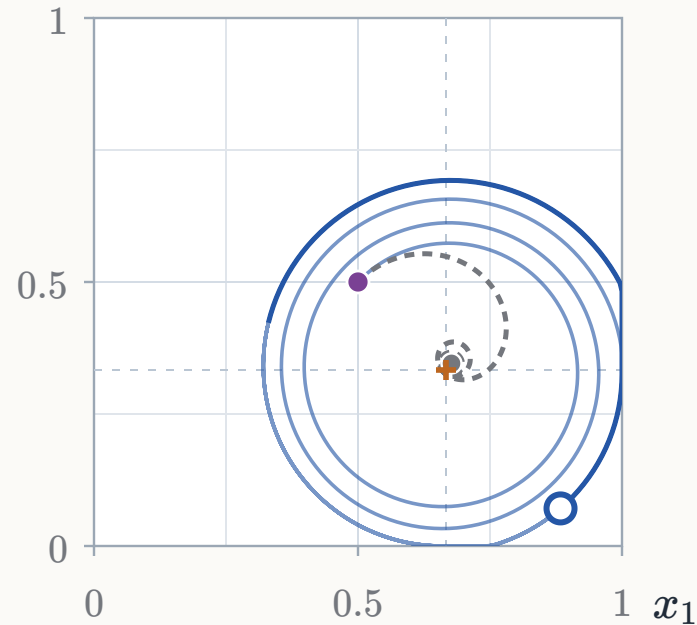
y_1 OGD
