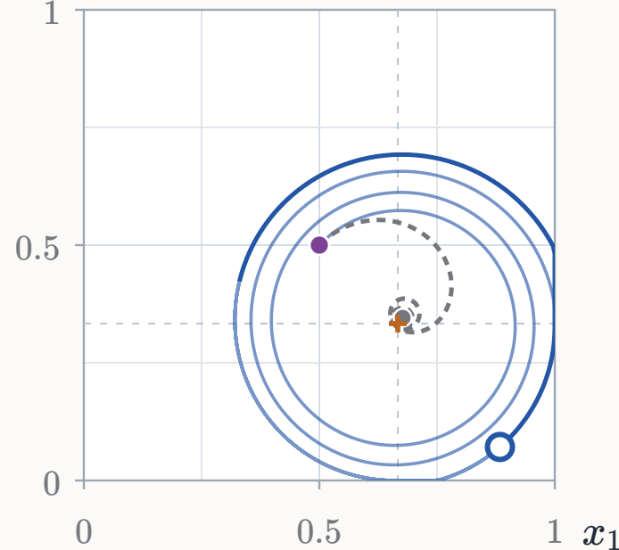
y_1 OGD
