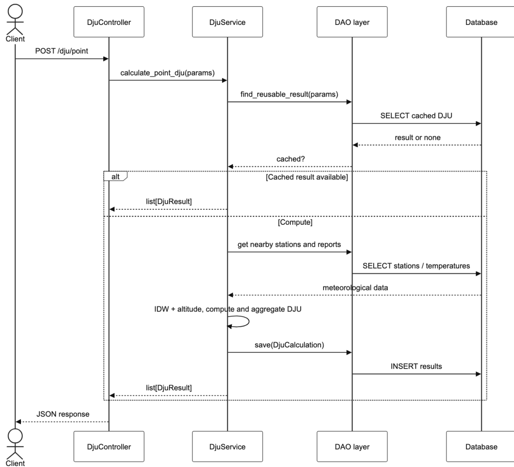
Figure 2.11 : Calcul d'un DJU ponctuel (F1)
