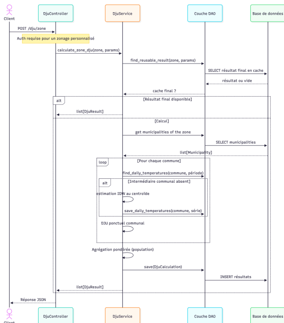
Figure A.6 : DJU zonal (F3)
