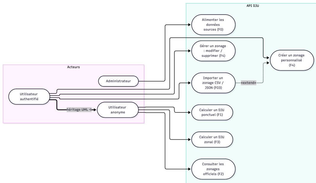
Figure 2.3 : Cas d'utilisation de l'API DJU
