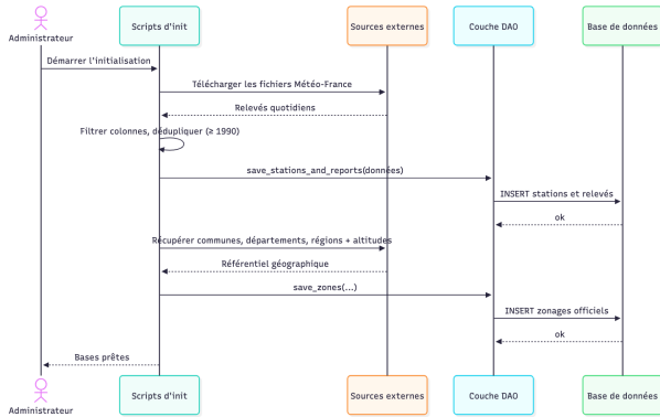
Figure A.4 : Initialisation (F0)
