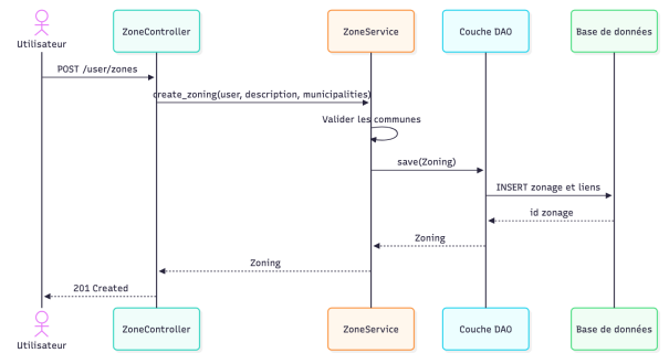
Figure A.9 : Création (F4)
