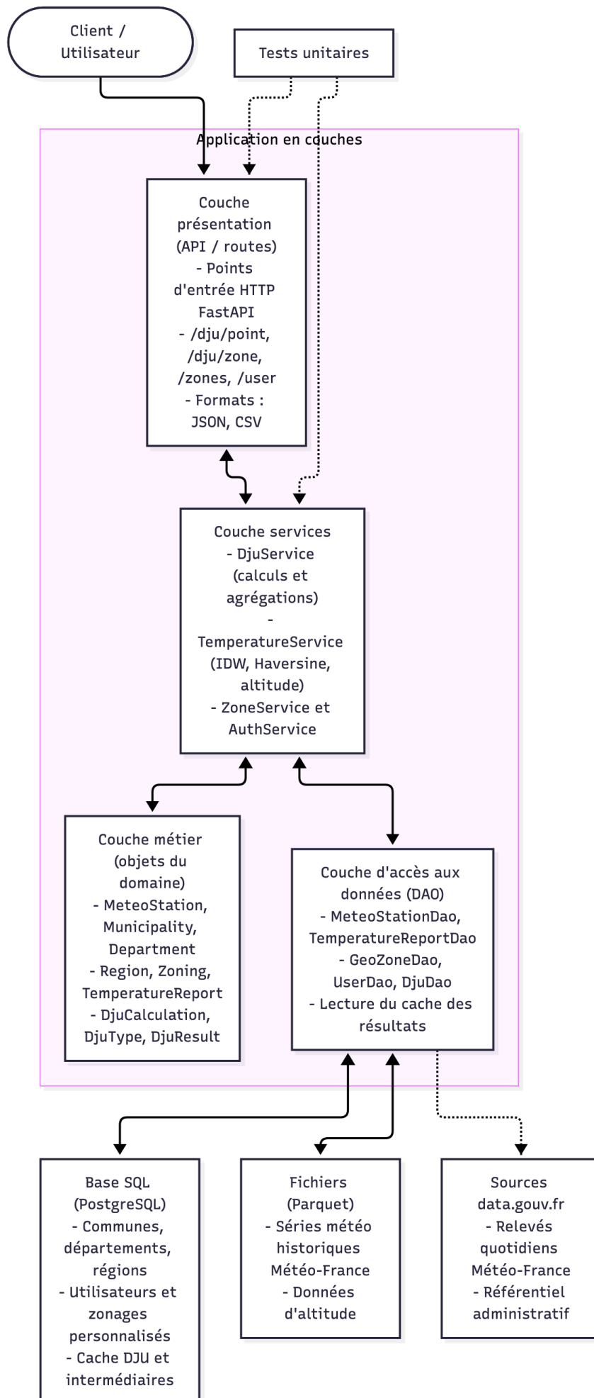
Figure 2.1 : Architecture en couches
