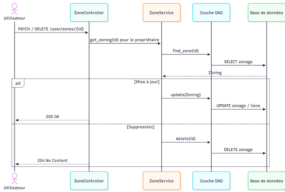
Figure A.10 : Gestion (F4)
