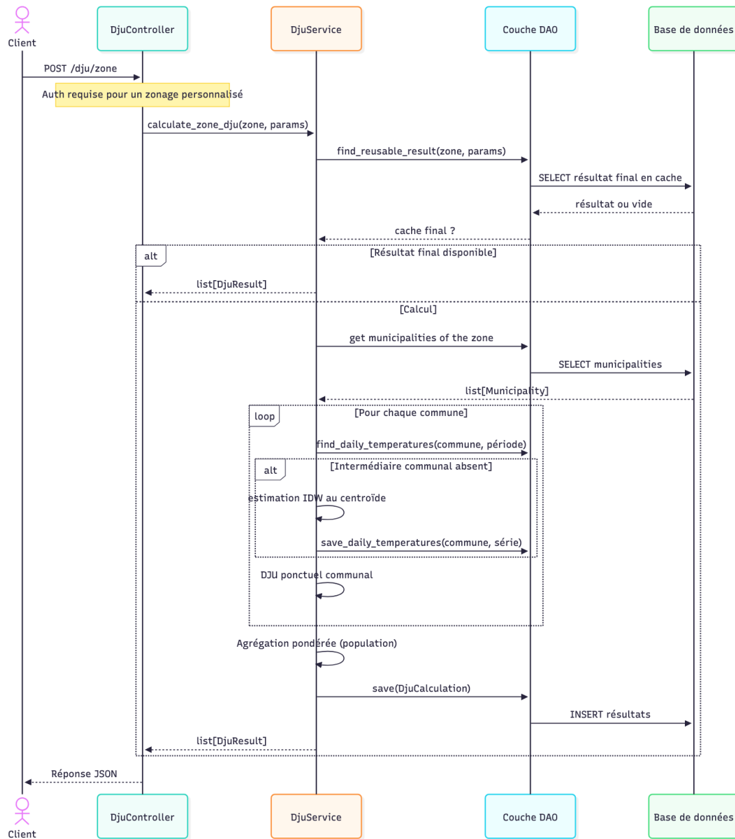
Figure 2.14 : Calcul d'un DJU zonal (F3)
