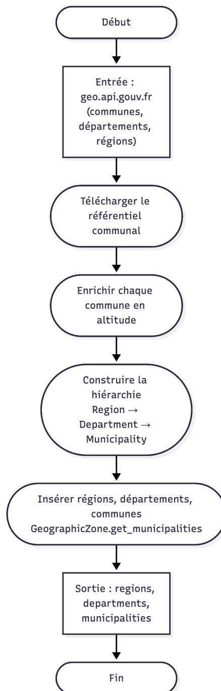
Figure 2.6 : Initialisation des zonages officiels
