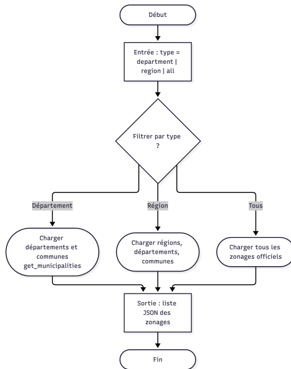
Figure 2.11 : Consultation des zonages officiels
