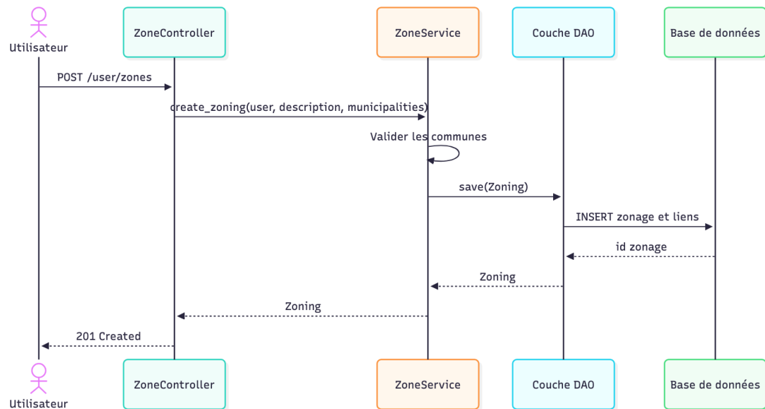
Figure 2.18 : Création d'un zonage personnalisé (F4)
