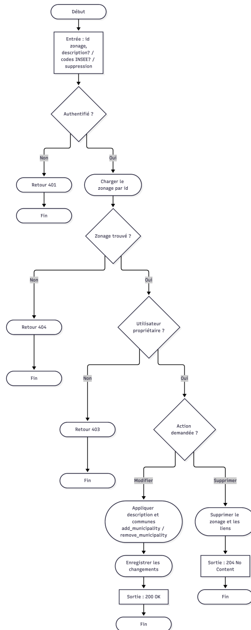
Figure 2.17 : Gestion d'un zonage personnalisé
