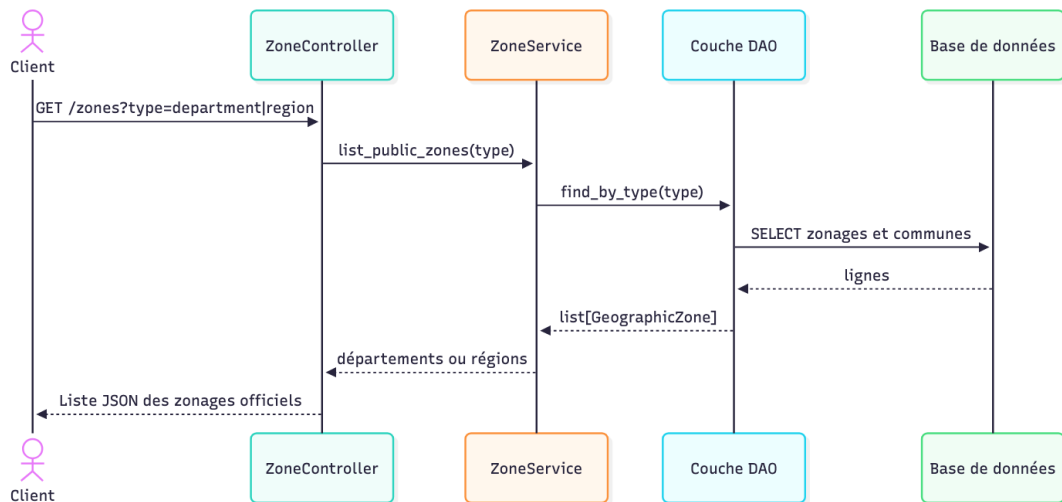
Figure 2.12 : Consultation des zonages publics (F2)
