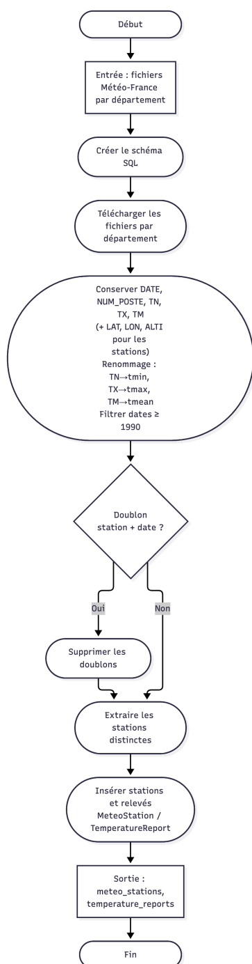
Figure 2.5 : Initialisation des stations et observations
