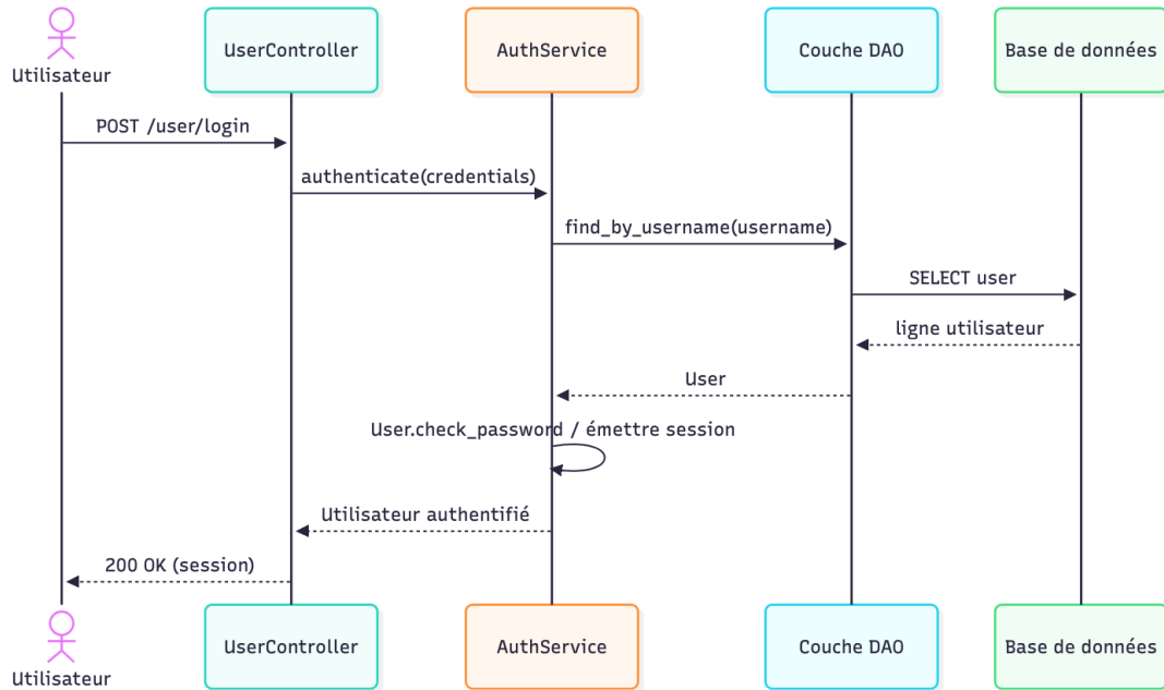
Figure 2.15 : Authentification d'un utilisateur
