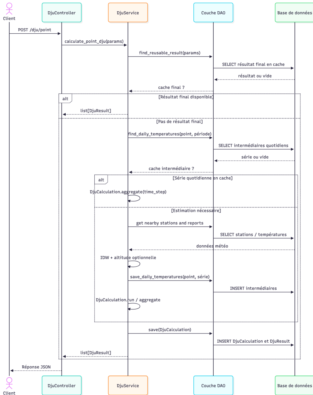
Figure 2.10 : Calcul d'un DJU ponctuel (F1)
