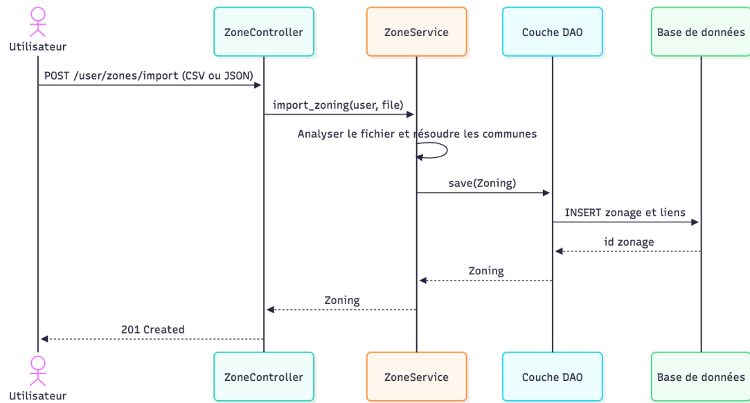
Figure 2.20 : Import d'un zonage depuis un fichier (FO3)
