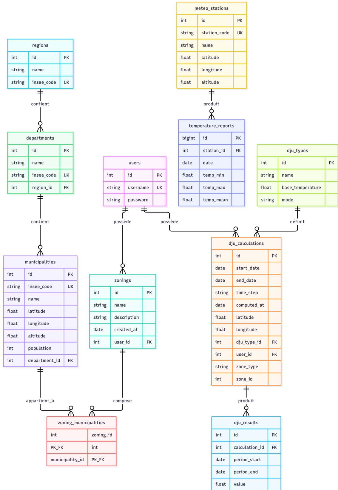
Figure 2.2 : Modèle entité-relation
