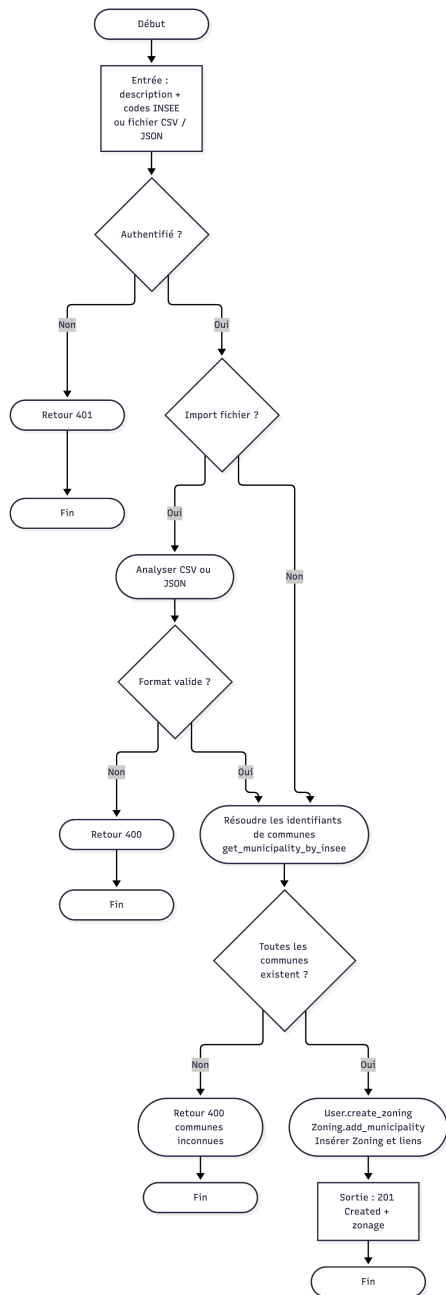
Figure 2.16 : Création ou import d'un zonage
