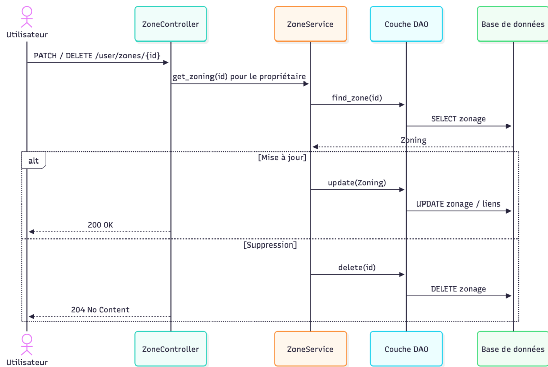
Figure 2.19 : Gestion d'un zonage personnalisé (F4)
