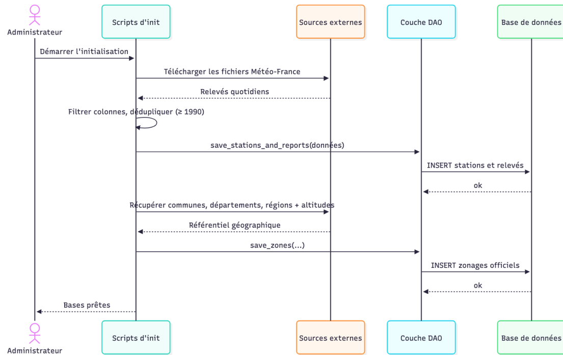
Figure 2.7 : Initialisation des bases de données (F0)
