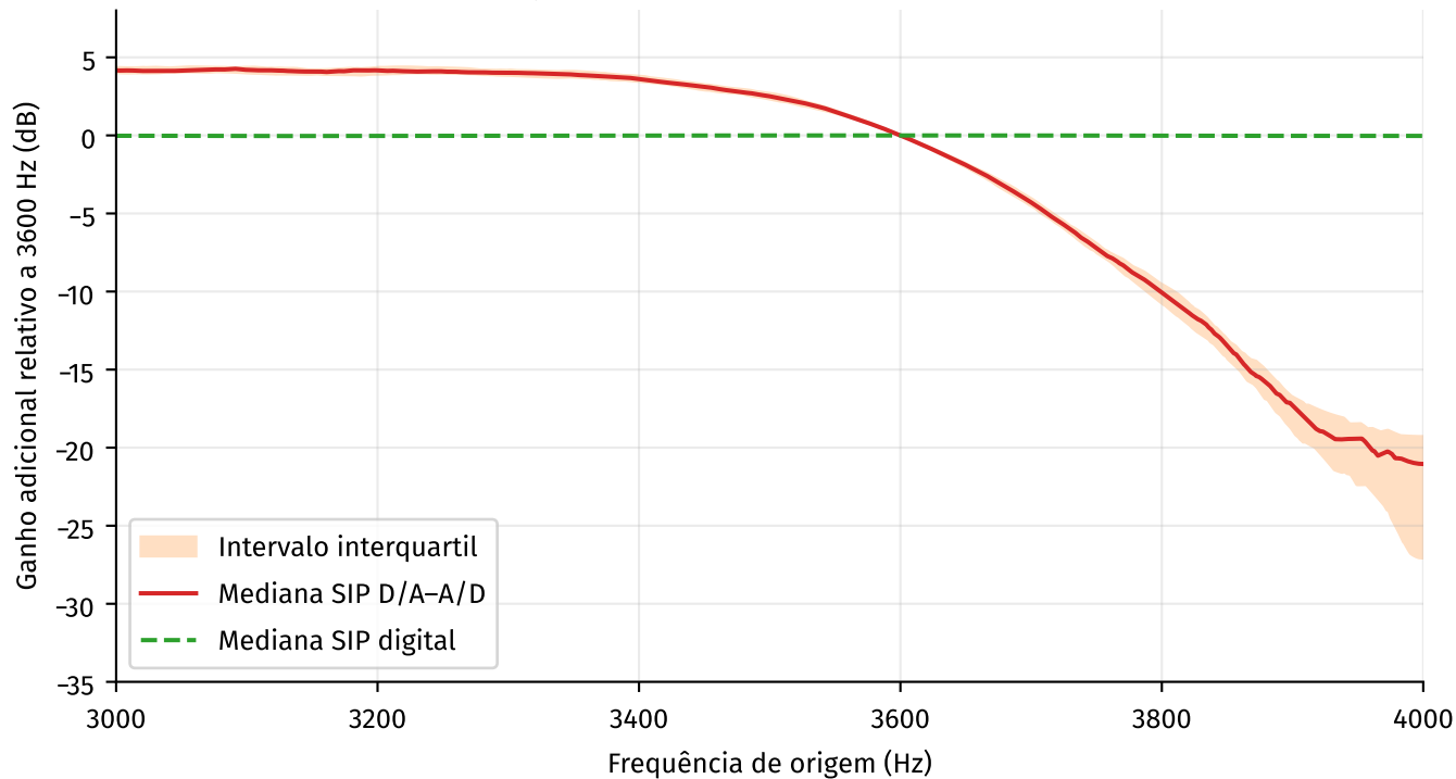
Resposta medida do caminho D/A-A/D
