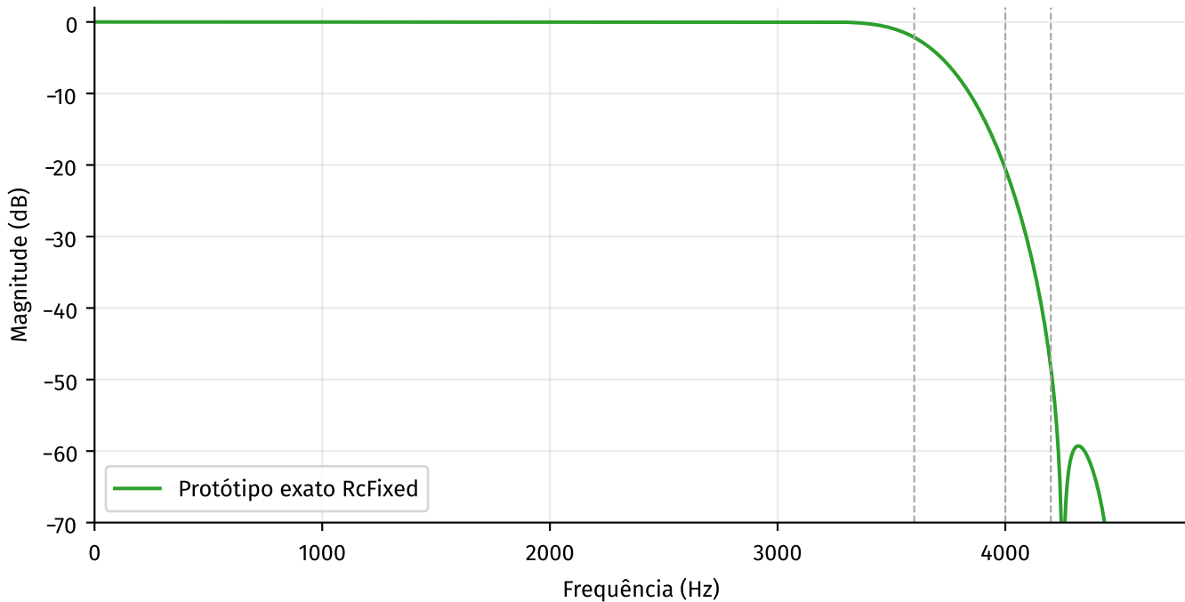
Resposta do RcFixed de 8,0 para 9,6 kamostras/s
