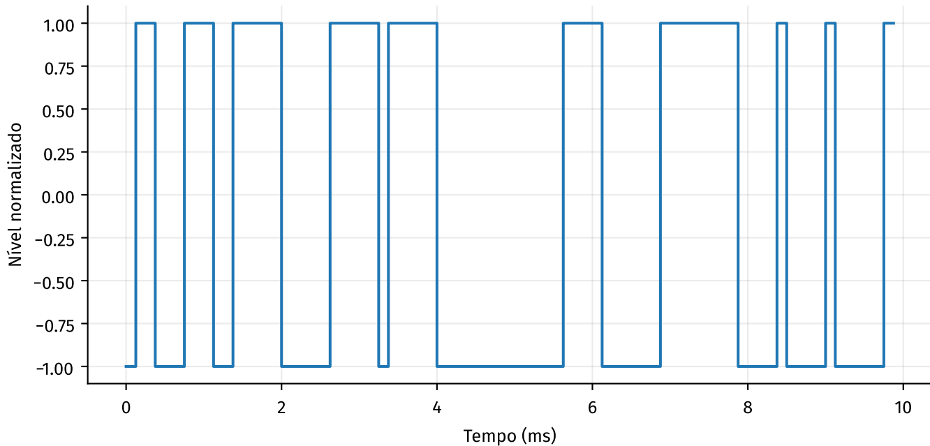
TRN1d capturada no E1: um símbolo antipodal por amostra a 8 kHz
