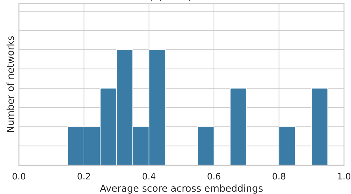
hcp | Group Lasso
