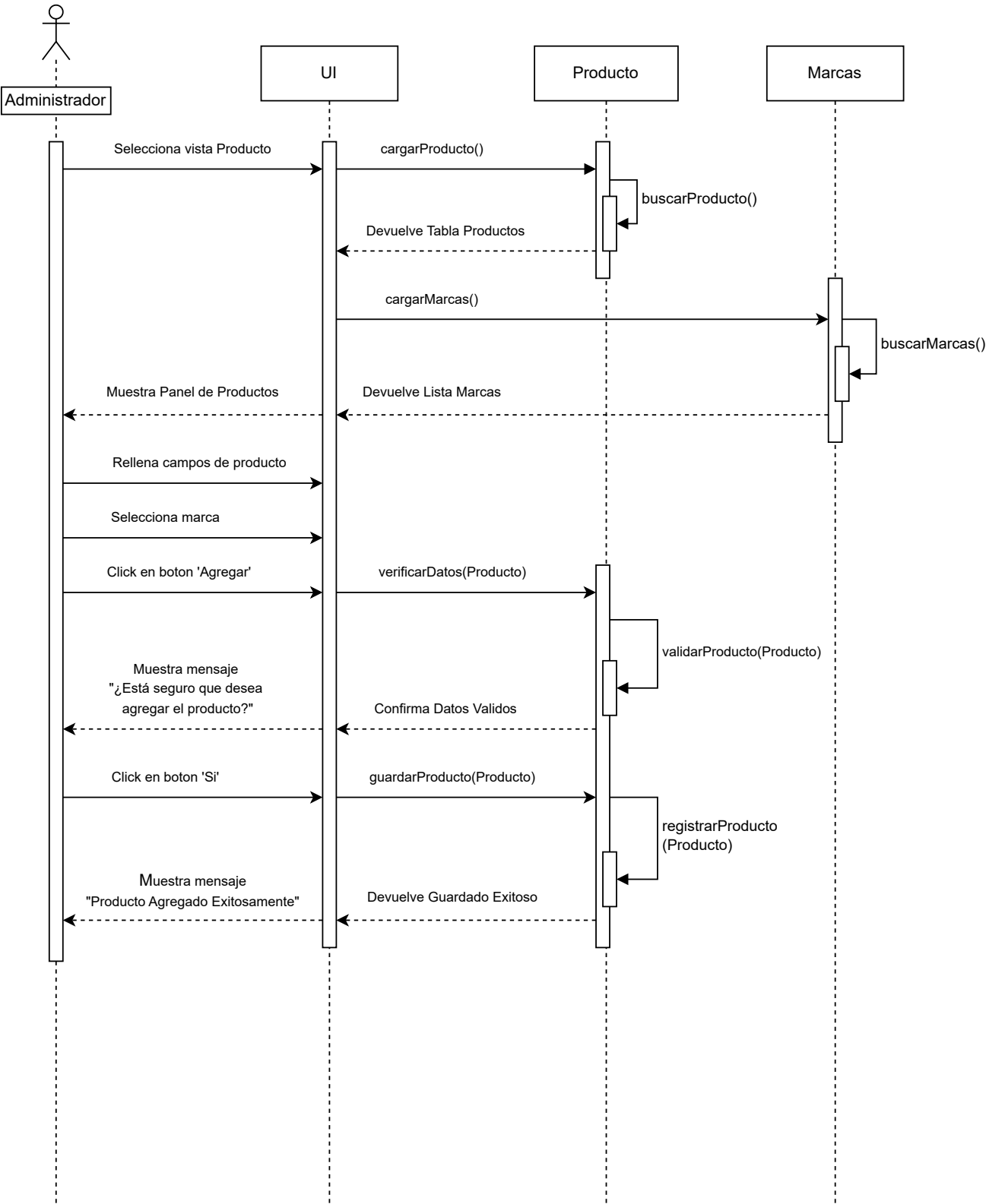
Diagrama de Secuencia, Administrador, agregar producto.
