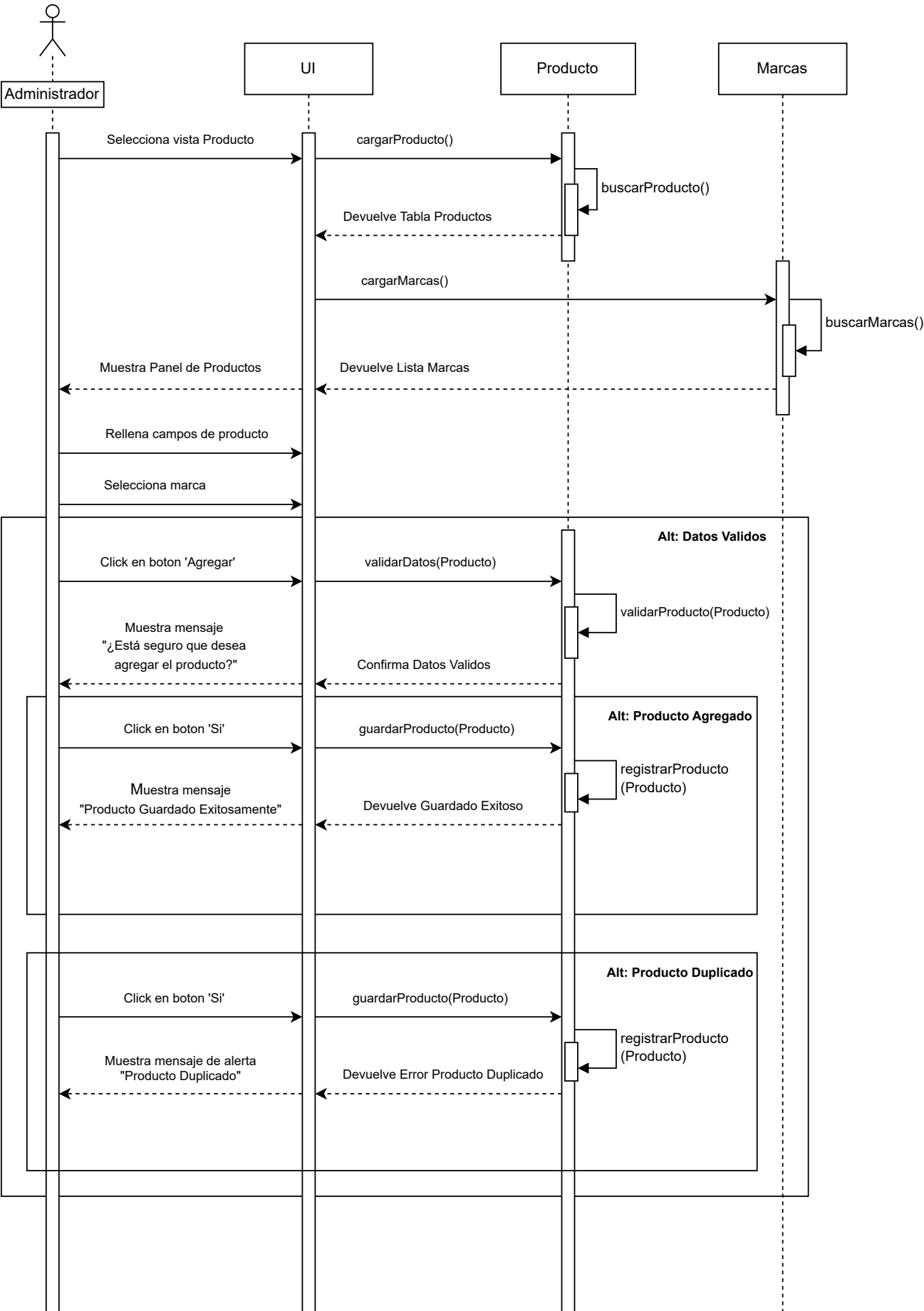
Diagrama de Secuencia, Administrador, agregar producto.
