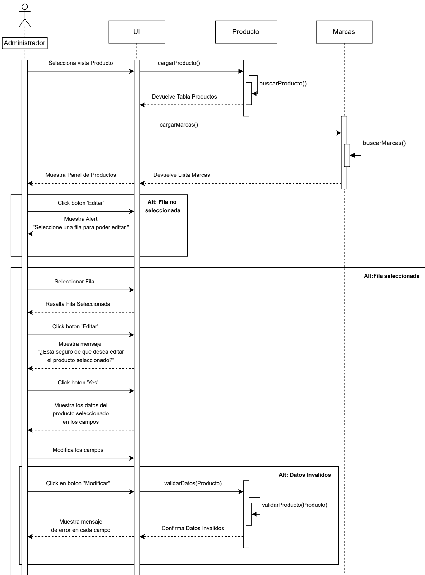
Diagrama de Secuencia, Administrador, modificar producto.
