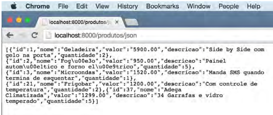
Fig. 9.7: Lista de produtos em formato JSON.
