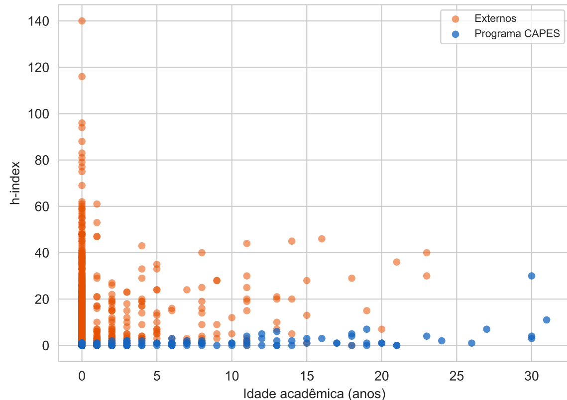
h-index vs Idade Acadêmica
