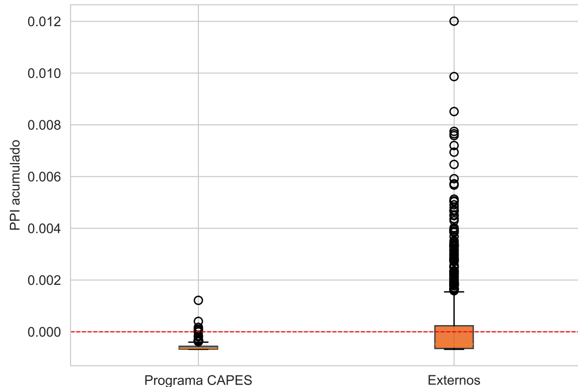
Dispersão (boxplot)
