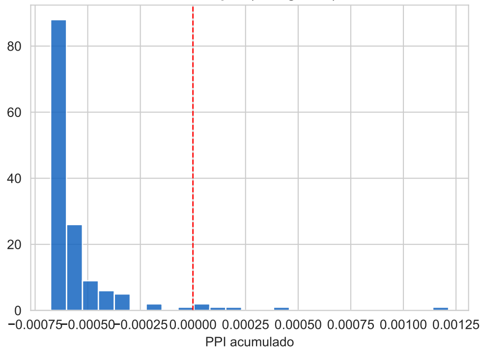
Distribuição (histograma)
