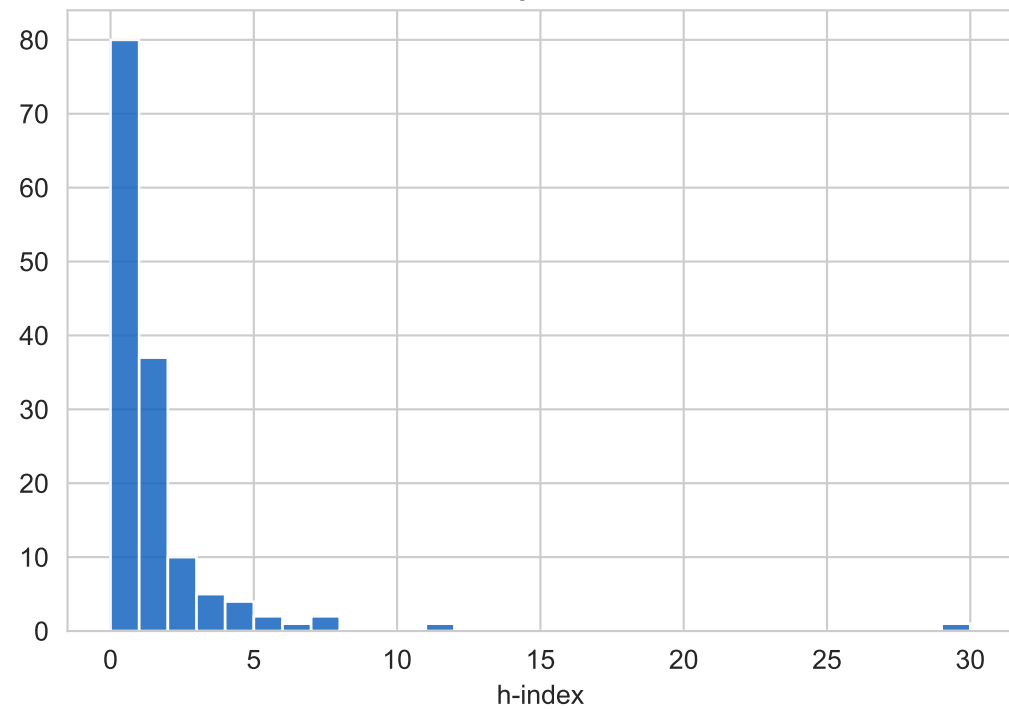
Distribuição h-index
