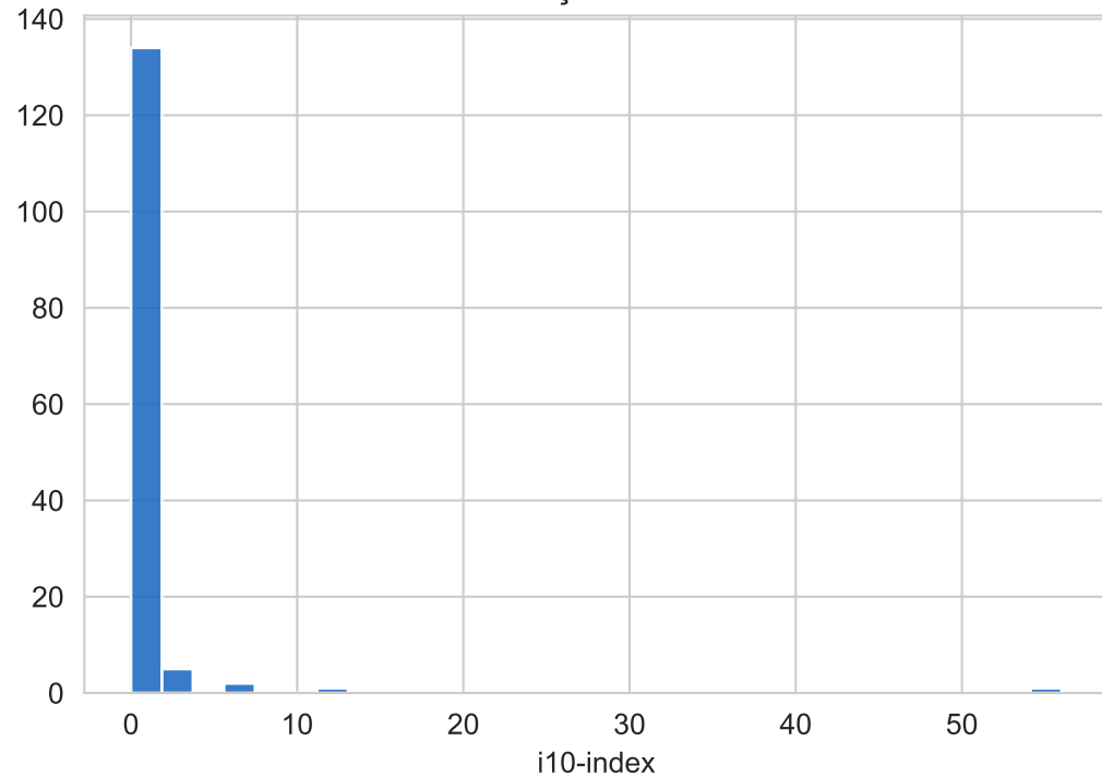
Distribuição i10-index
