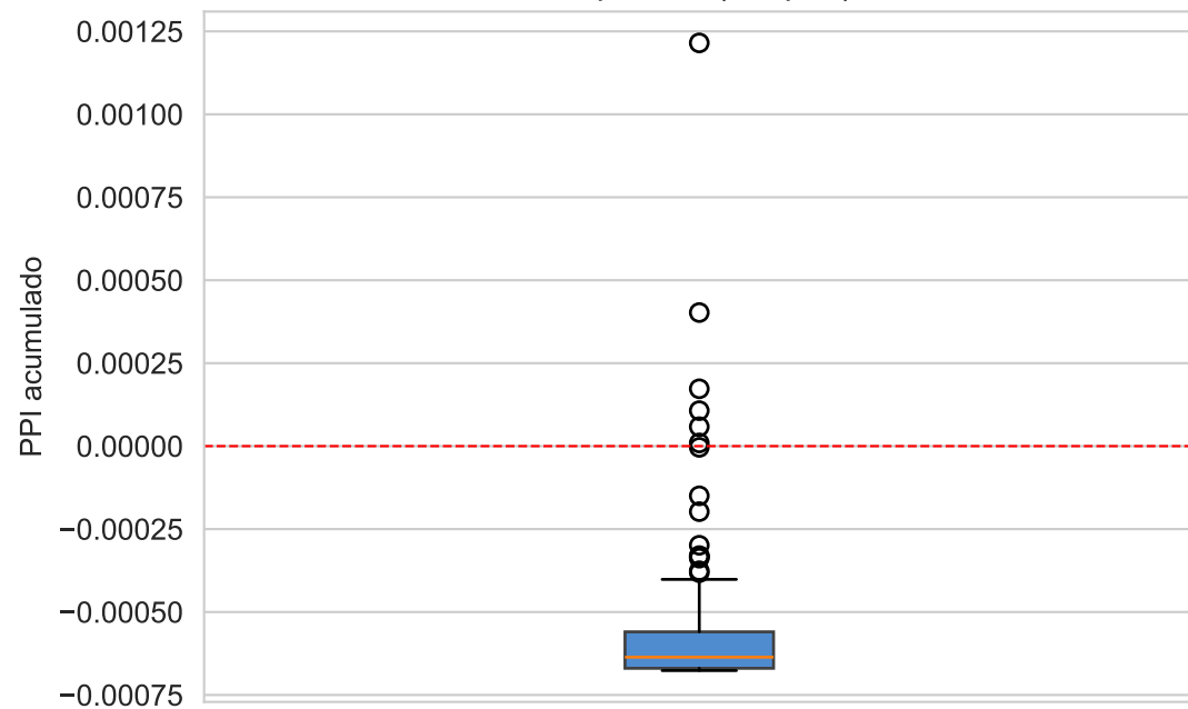
Dispersão (boxplot)
