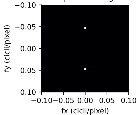
due picchi coniugati
