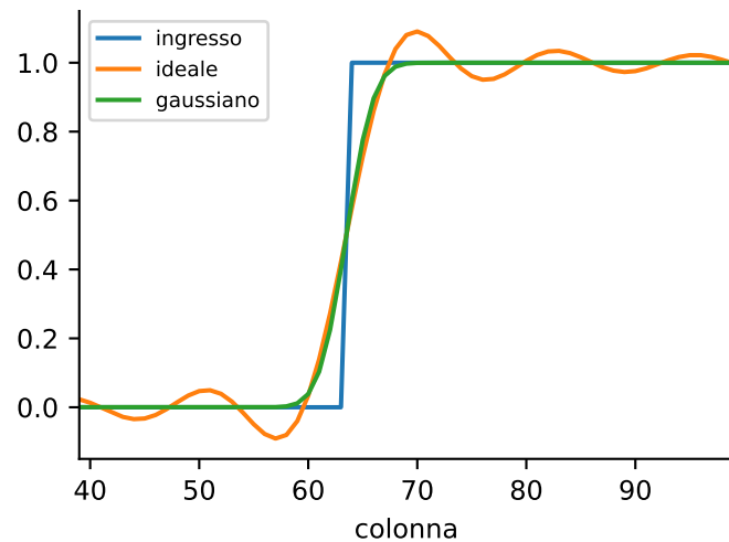
risposta a un bordo
