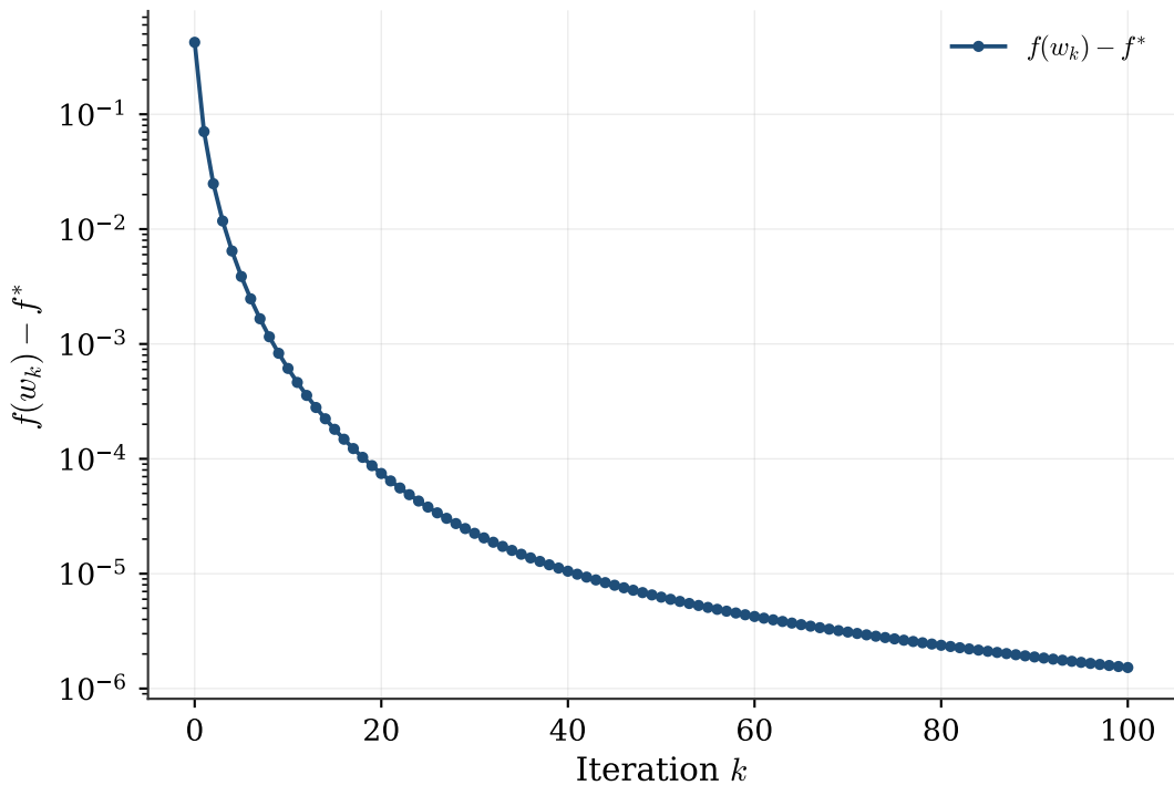
IRLS
