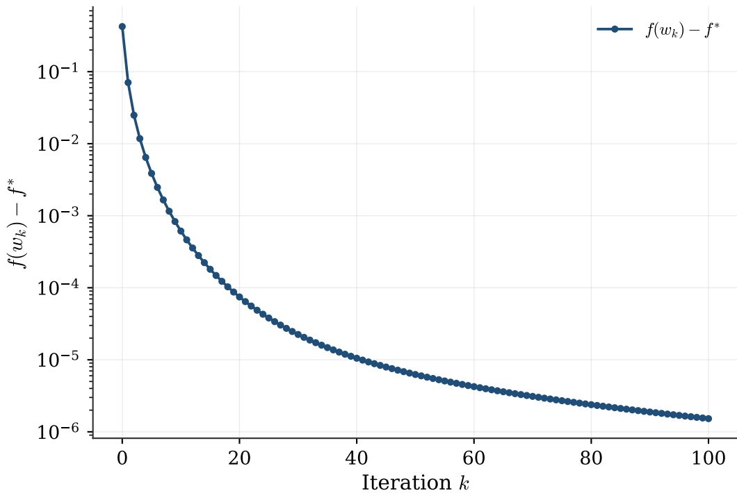
IRLS
