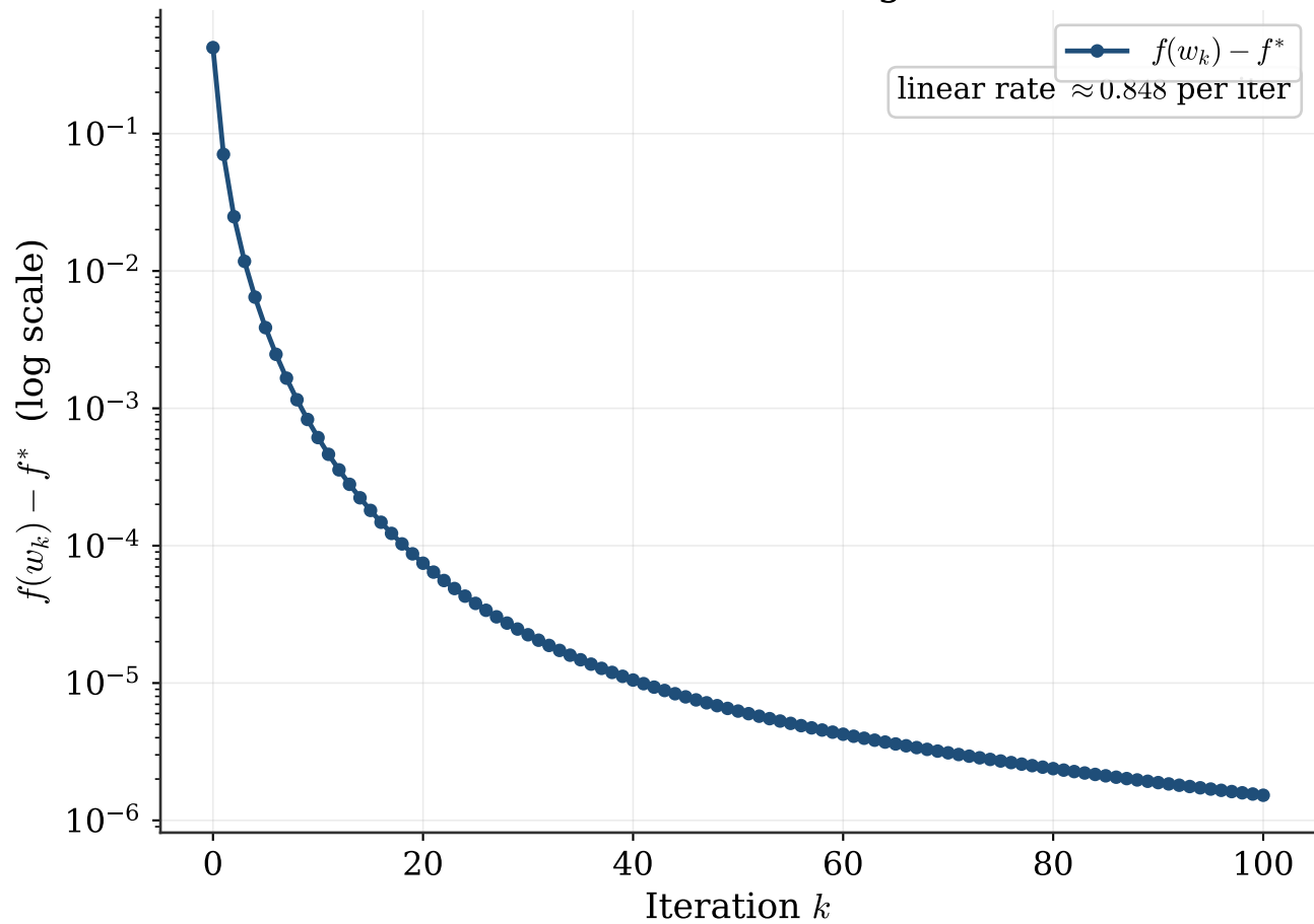
IRLS: linear convergence
