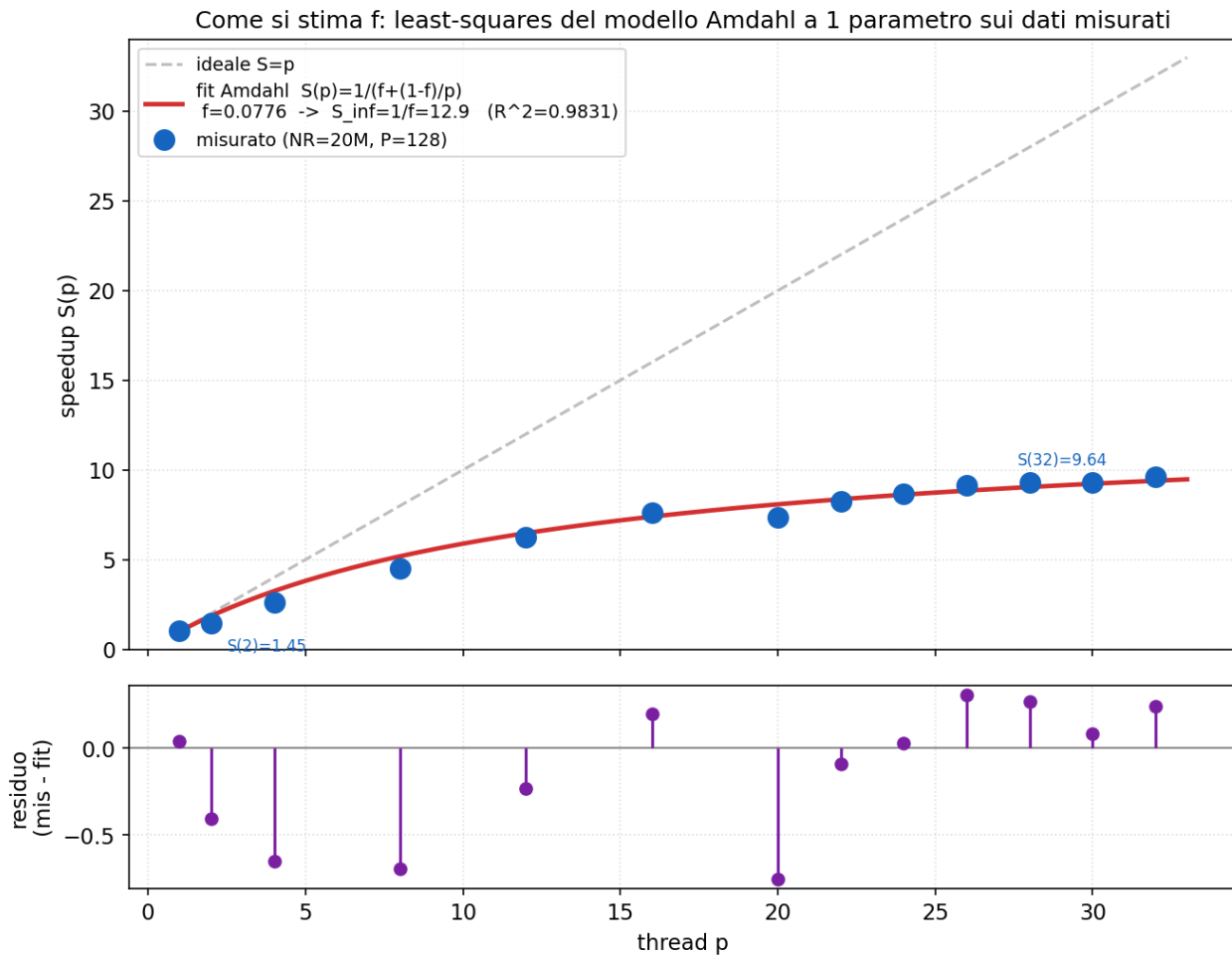
Figure 13: Come si stima f: least-squares del modello Amdahl sui dati misurati, con residui e R^2 .
