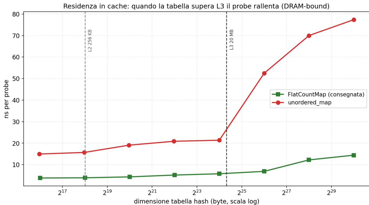
Figure 6: Residenza in cache: quando la tabella supera L3 il probe rallenta (DRAM-bound).
