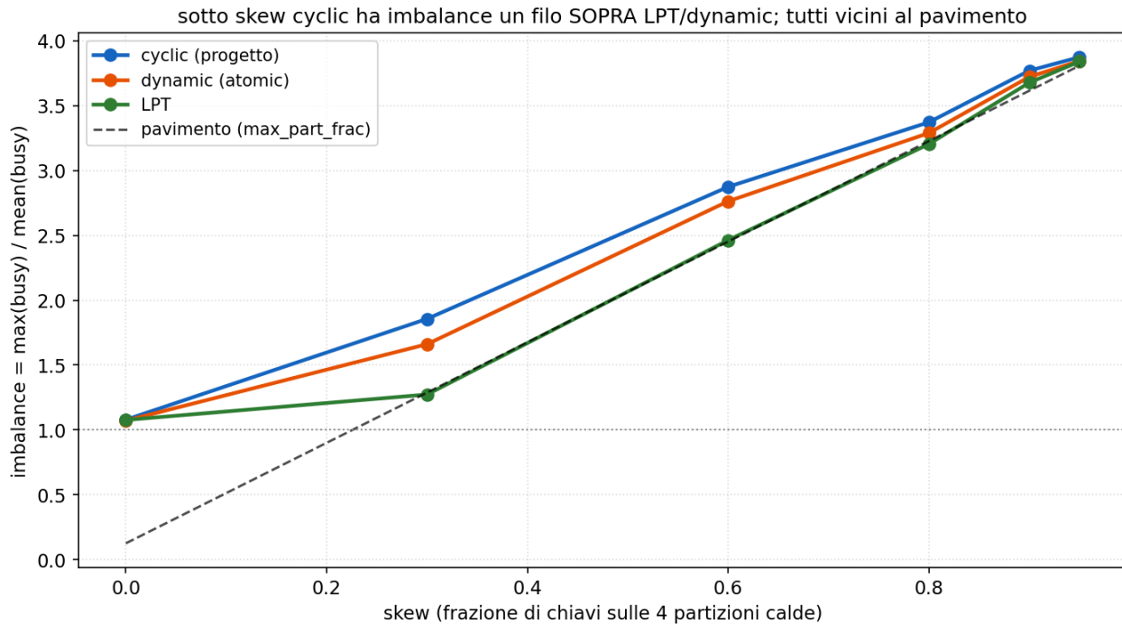
Figure 10: Sotto skew l'imbalance di cyclic sta un filo SOPRA LPT/dynamic; tutti vicini al pavimento (nessuno lo batte).
