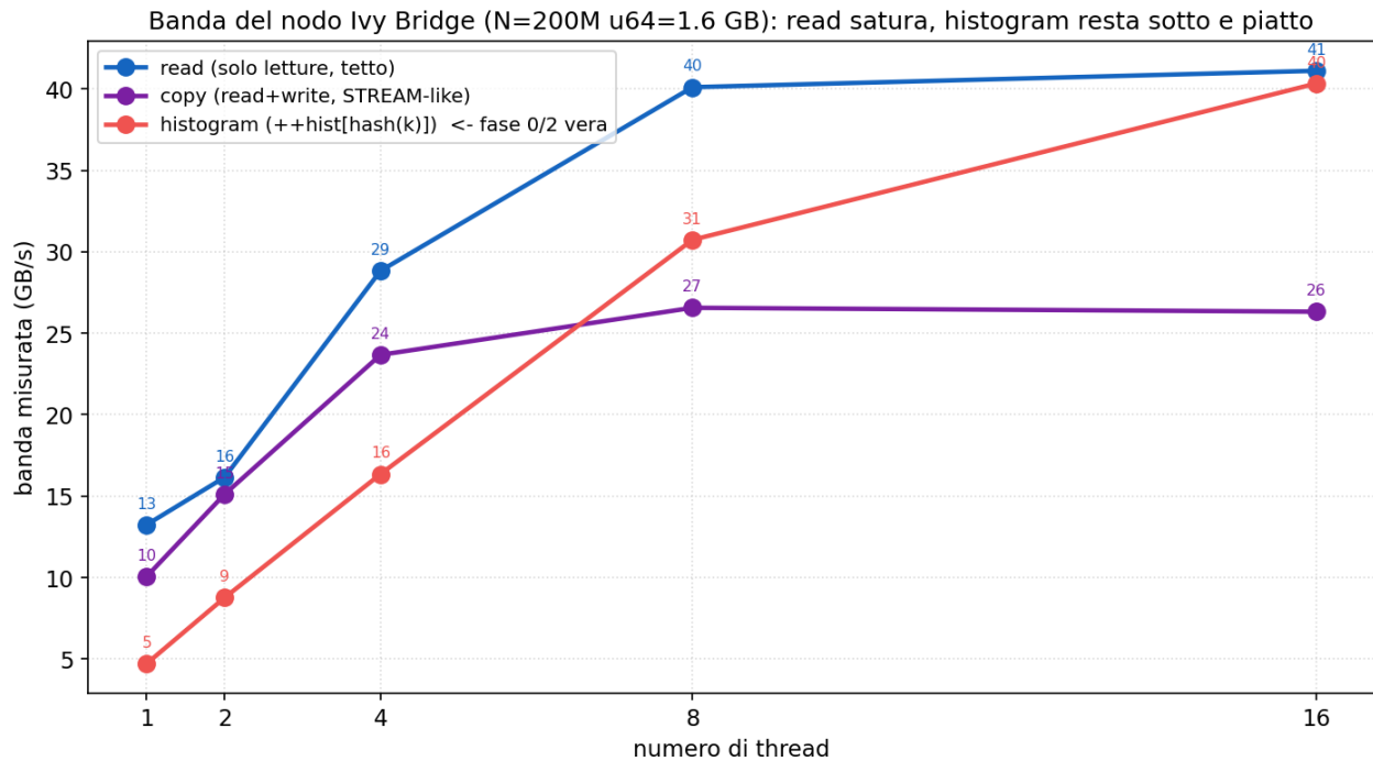
Figure 11: Banda del nodo: read saturo a ~41 GB/s, l'histogram raggiunge lo stesso tetto a 16 core.
