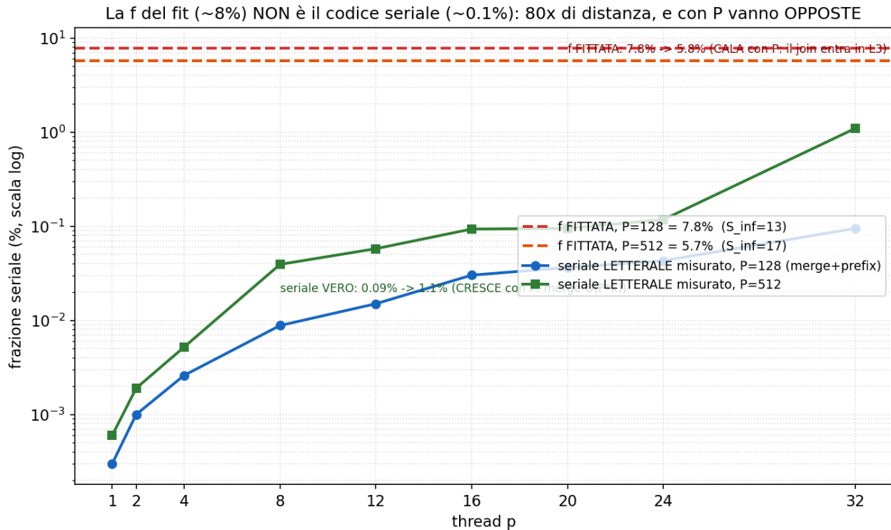
Figure 14: La f del fit (~8%) NON è il codice seriale (~0.1%): 80x di distanza, e con P vanno OPPOSITE.
