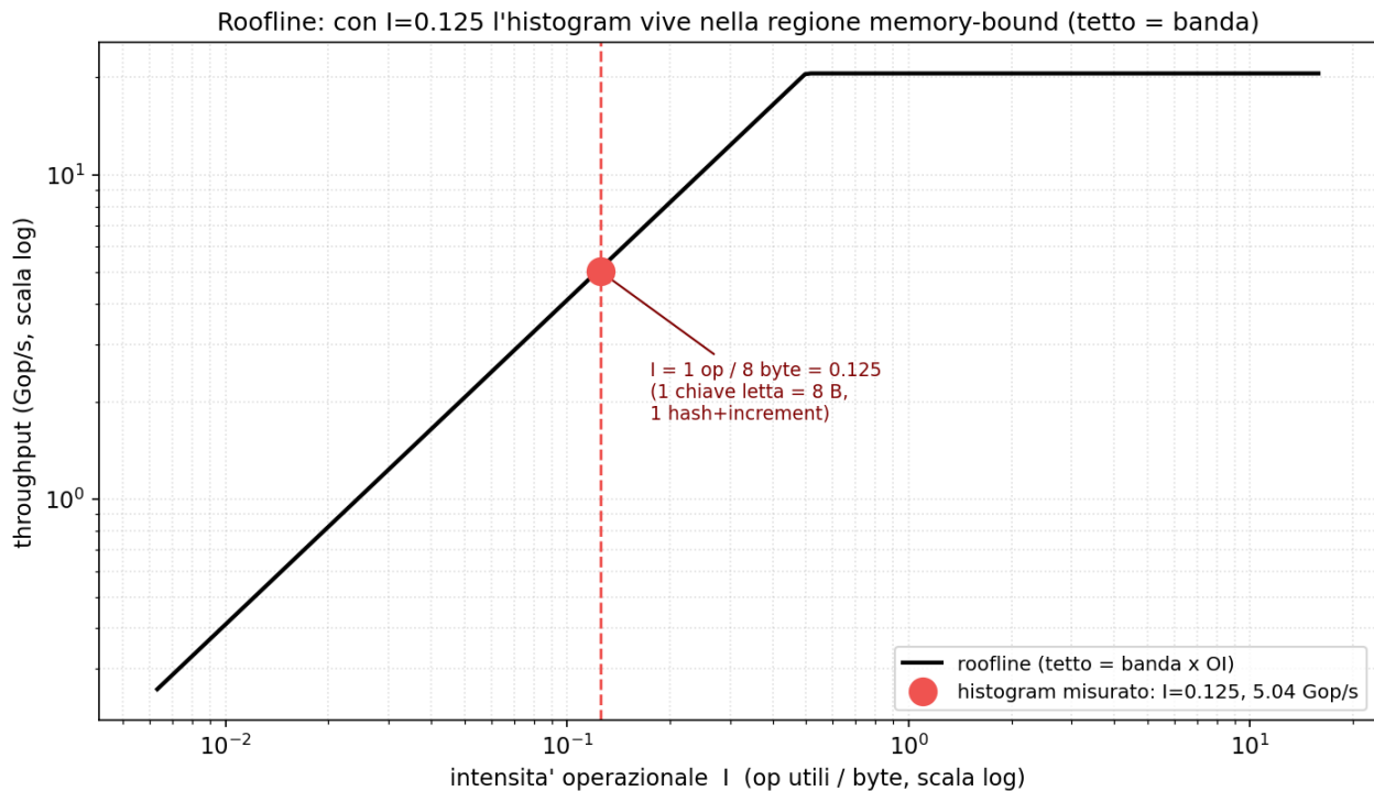
Figure 12: Roofline: con I=0.125 l'histogram vive nella regione memory-bound (tetto = banda).
