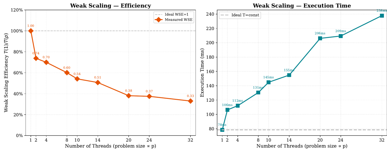
Figure 17: Report: weak scaling, efficienza (sinistra) e tempo assoluto (destra).
