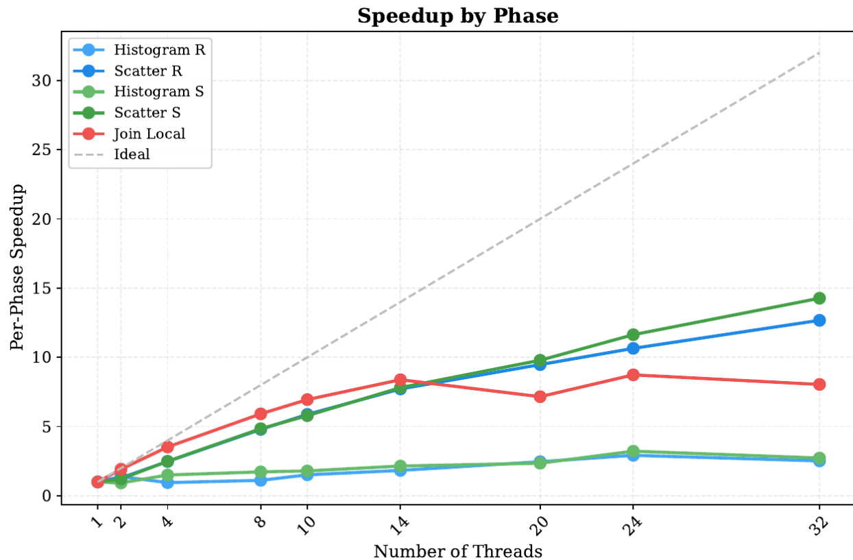
Figure 16: Report: speedup per fase. Scatter sale anche in HT, Histogram resta piatto, Join fa plateau.
