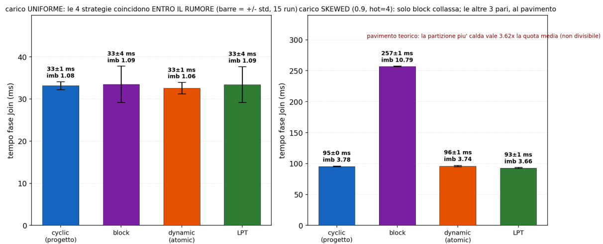
Figure 9: Uniforme: le 4 strategie coincidono entro il rumore. Skew: solo block collassa; le altre 3 pari, al pavimento.
