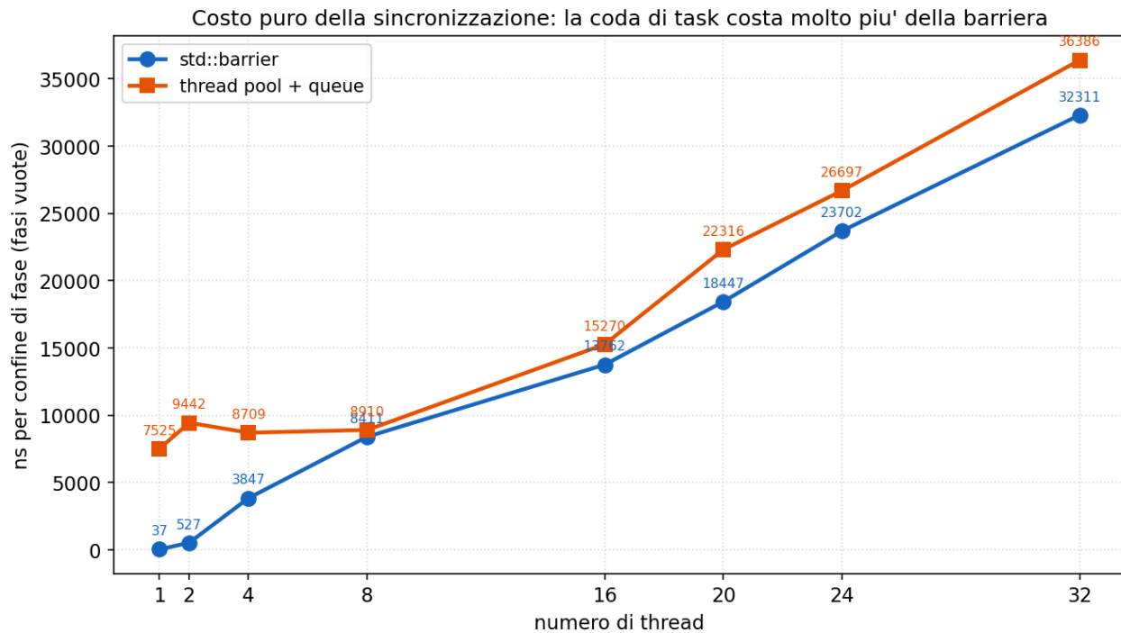
Figure 8: Costo puro di un confine di fase: la coda di task costa molto piu' della barriera.
