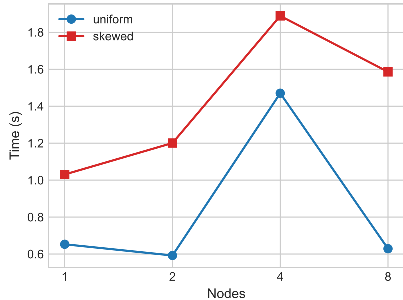
Pure MPI
