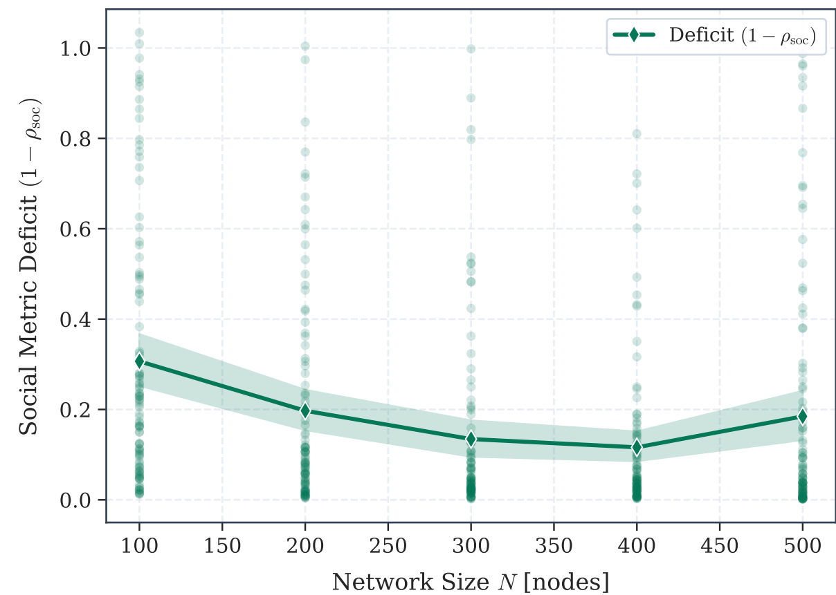
(d) Latent Social Metric Space Recovery
