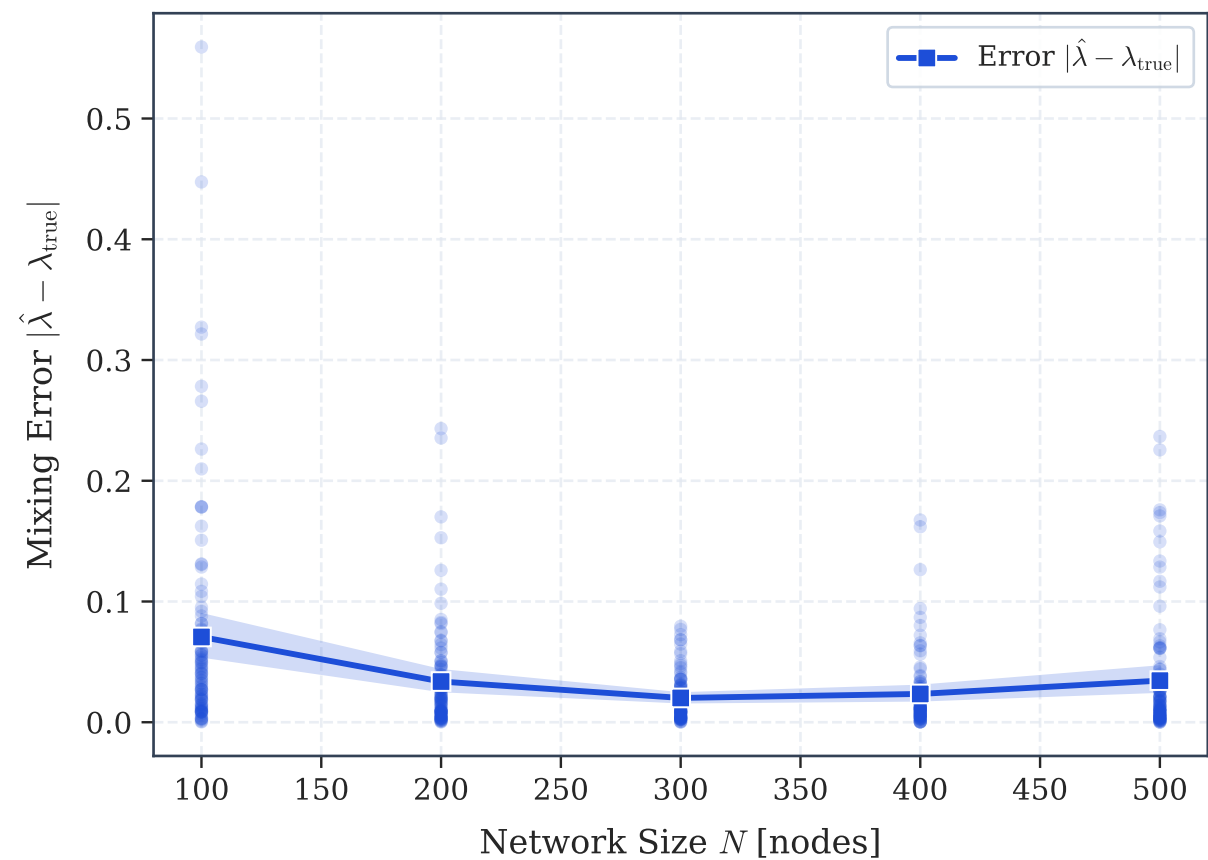
(b) Mixing Parameter Estimation Error
