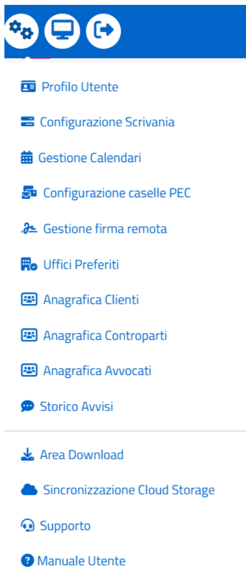
Figura 10 - Profilo Utente e Configurazioni
