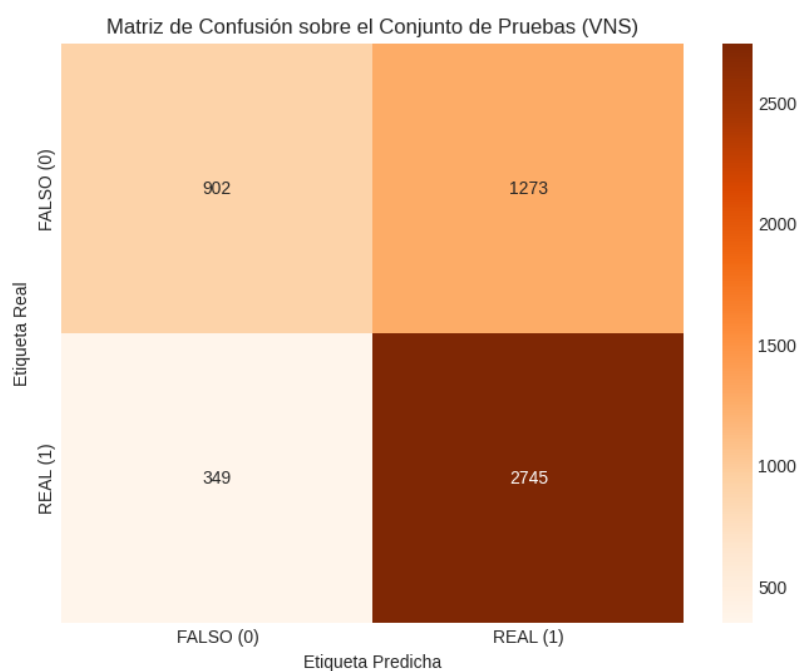
Figura 5.9: Matriz de confusión para VNS destacando la excelente exhaustividad del 89 % para detección de noticias reales con especificidad competitiva del 41 %.
