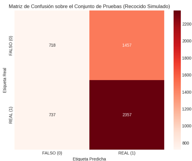
Figura 5.3: Matriz de confusión para MSA en el conjunto de pruebas, evidenciando la baja especificidad (33 %) y el sesgo hacia la clasificación como noticias reales.
