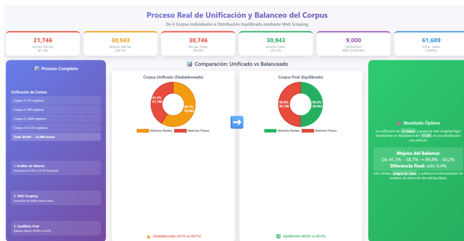
Figura 4.2: Representación gráfica del proceso de balanceo del corpus: comparación entre distribución inicial desbalanceada y distribución final equilibrada. La imagen muestra cómo la extracción web de 9,000 noticias falsas permitió alcanzar un equilibrio óptimo de 49.8 % noticias falsas vs 50.2 % noticias reales.
