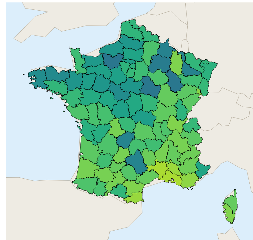
a Precision
