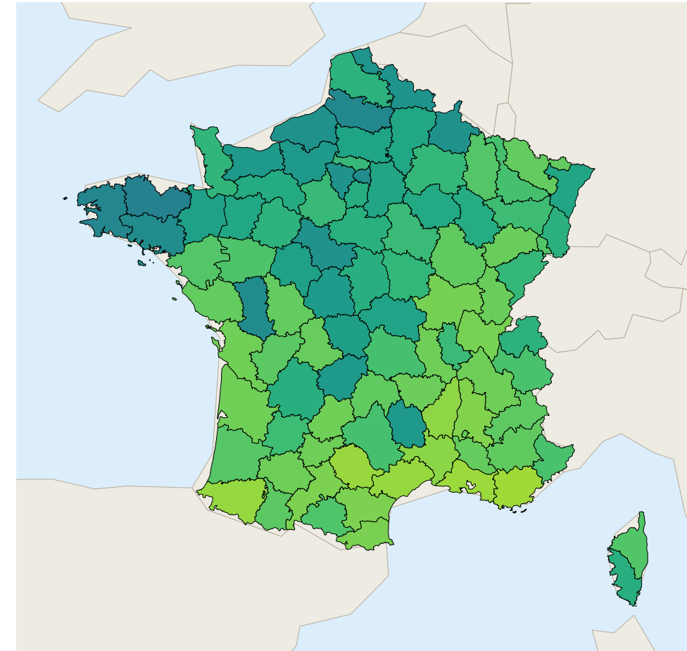
F1
