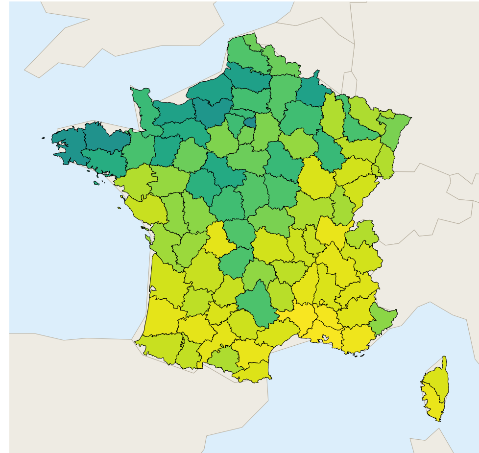
Precision
