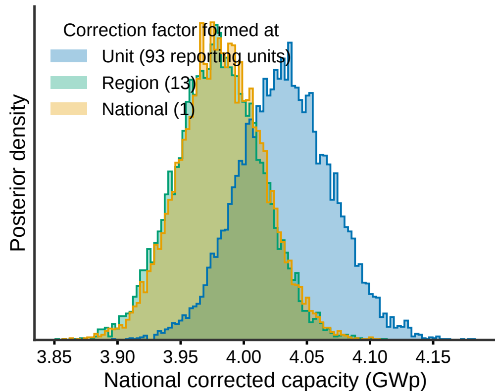
a Posterior of the national total
