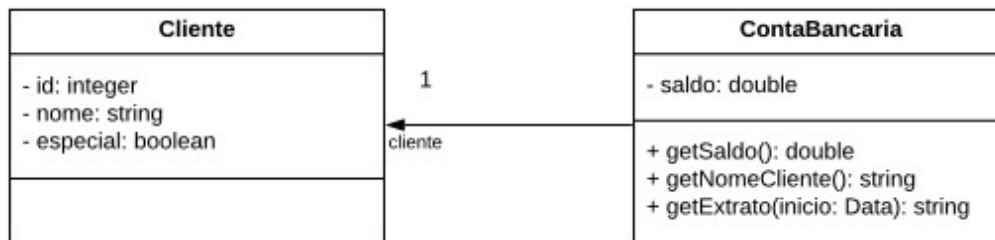
Exemplo de Diagrama de Classe UML
