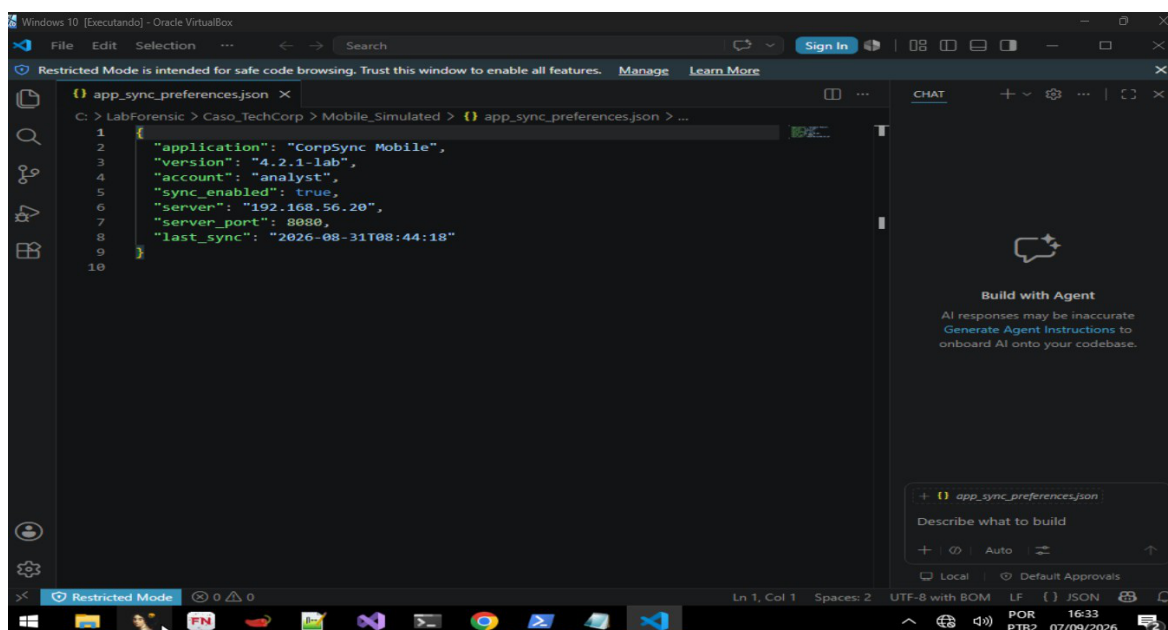
Figura 4 – Configuração do aplicativo móvel em app_sync_preferences.json
