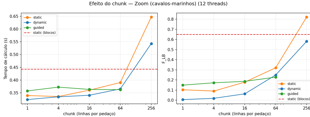
Figura 7 — Efeito do tamanho do chunk sobre o tempo de cálculo e o Fator de Balanceamento de Carga no zoom.
