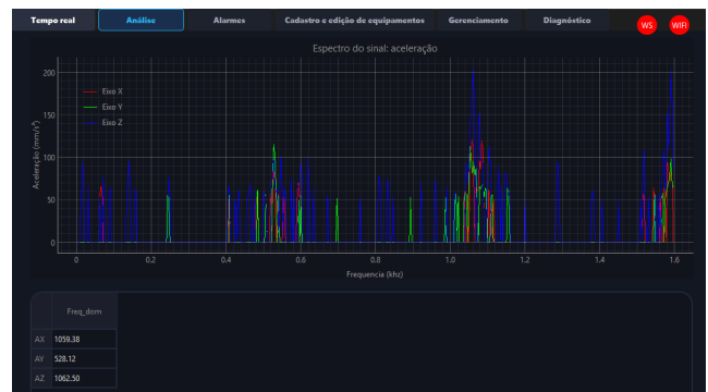
Fig. 10. MIT sem perturbação: FFT do sinal de aceleração.
