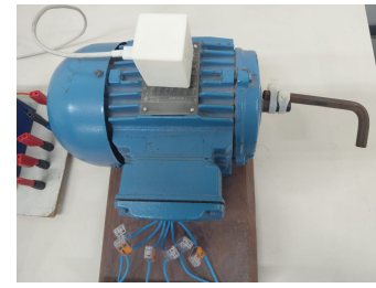
Fig. 13. Perturbação induzida no MIT por meio de carga desbalanceadora.
