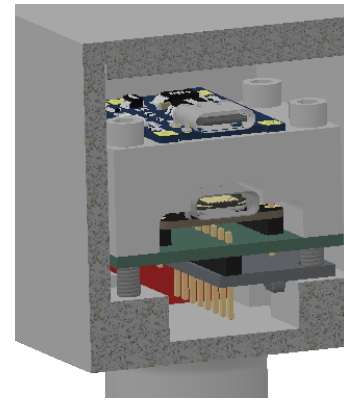
Fig. 3. Vista em corte do dispositivo desenvolvido. Fonte: Elaborado pelo autor.
