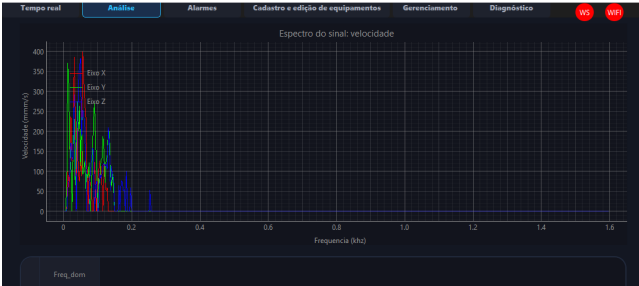
Fig. 21. MIT com impacto: FFT do sinal de velocidade. Fonte: Elaborado pelo autor.
