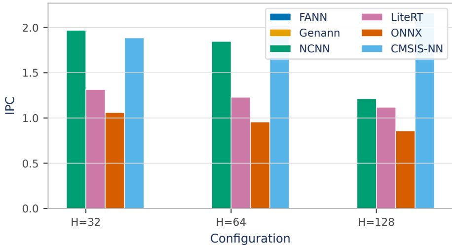
IPC — LSTM
