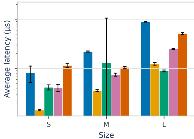
Sigmoid
